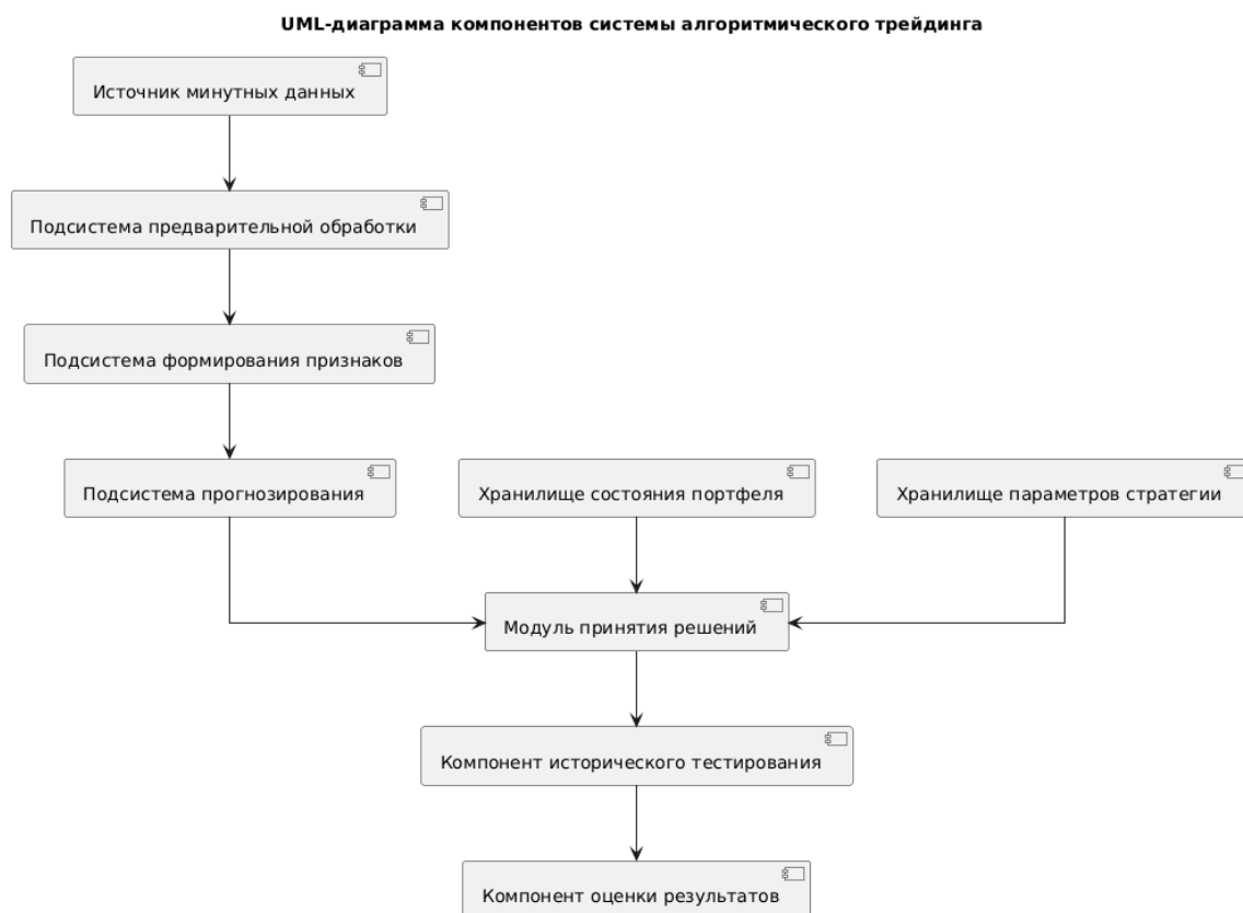
Рисунок 1 – Диаграмма компонентов системы алгоритмического трейдинга
