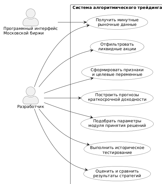
Рисунок 3 – Диаграмма вариантов использования системы трейдинга
