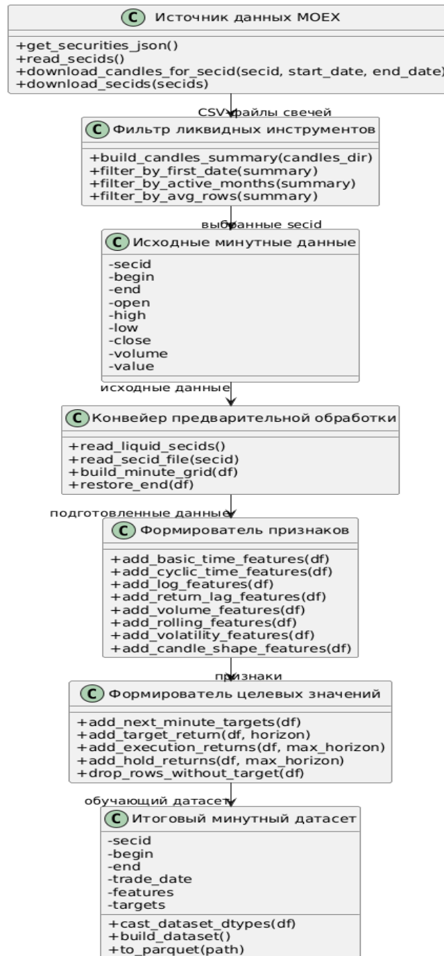
UML-диаграмма классов подсистемы подготовки данных
