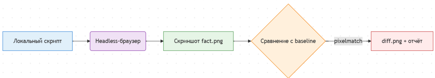
Рисунок 3 — Схема работы open-source инструментов попиксельного сравнения
