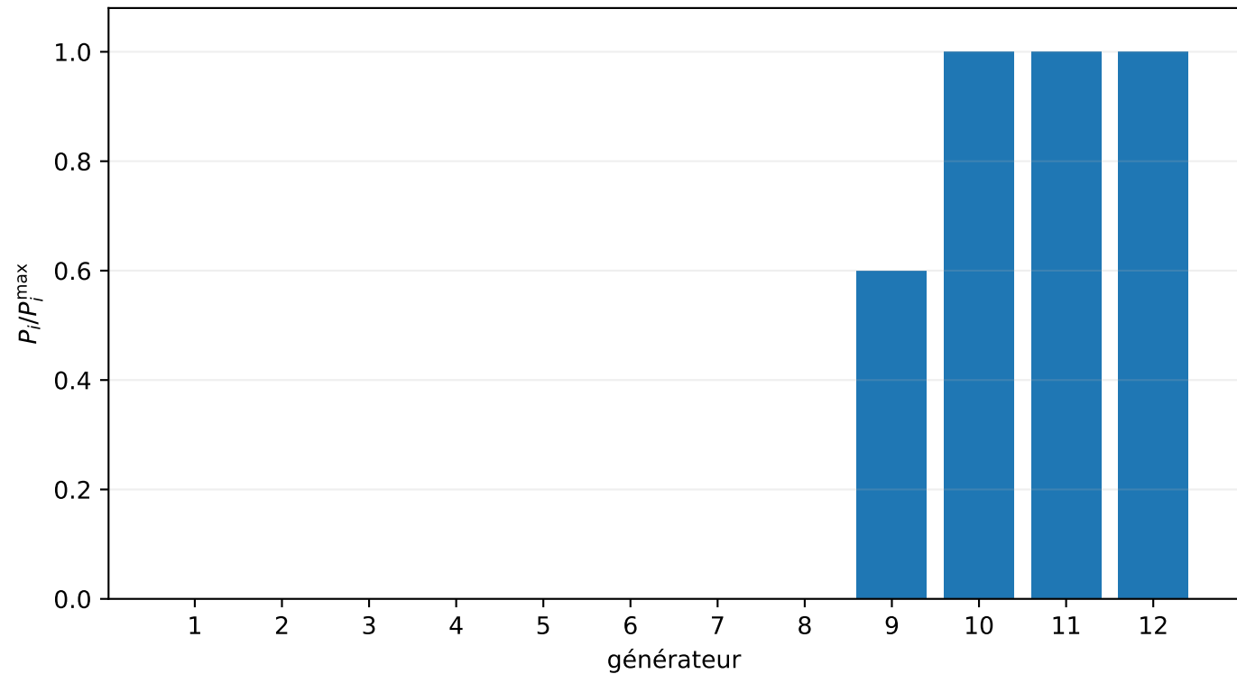
Répartition de la production entre les 12 générateurs — P_D/P_C = 0.300
