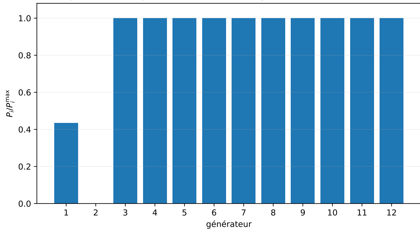
Répartition de la production entre les 12 générateurs — P_D/P_C = 0.870
