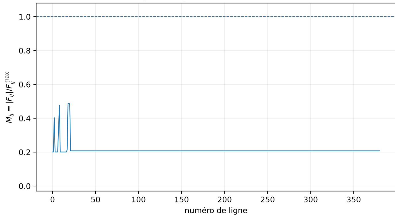
Fraction de charge des lignes à faible demande — P_D/P_C = 0.300
