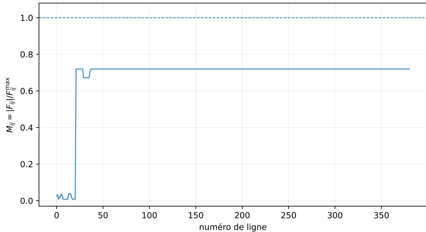
Lignes juste au-dessus de la limite de génération — P_D/P_C = 1.040
