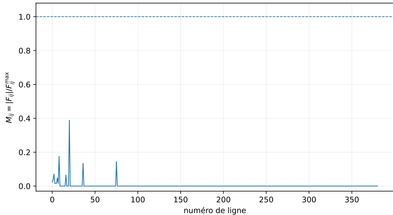
Lignes au voisinage de la limite de transport — P_D/P_C = 1.450
