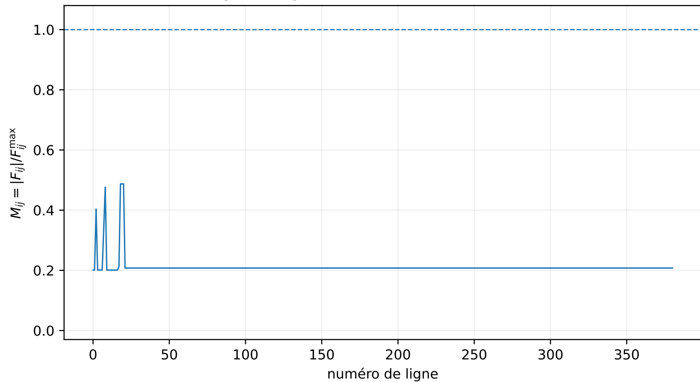
Fraction de charge des lignes à faible demande — P_D/P_C = 0.300 (initial)
