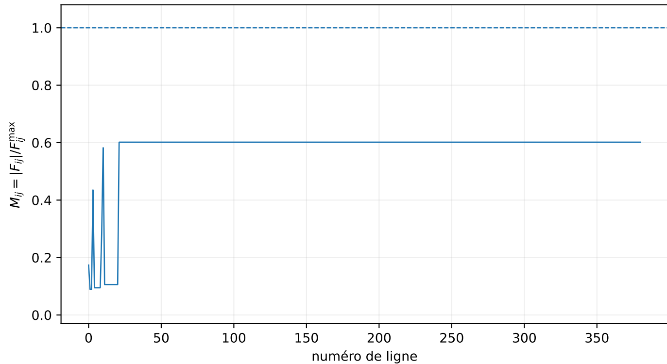
Fraction de charge des lignes — charges de la Table I — P_D/P_C = 0.870 (initial)
