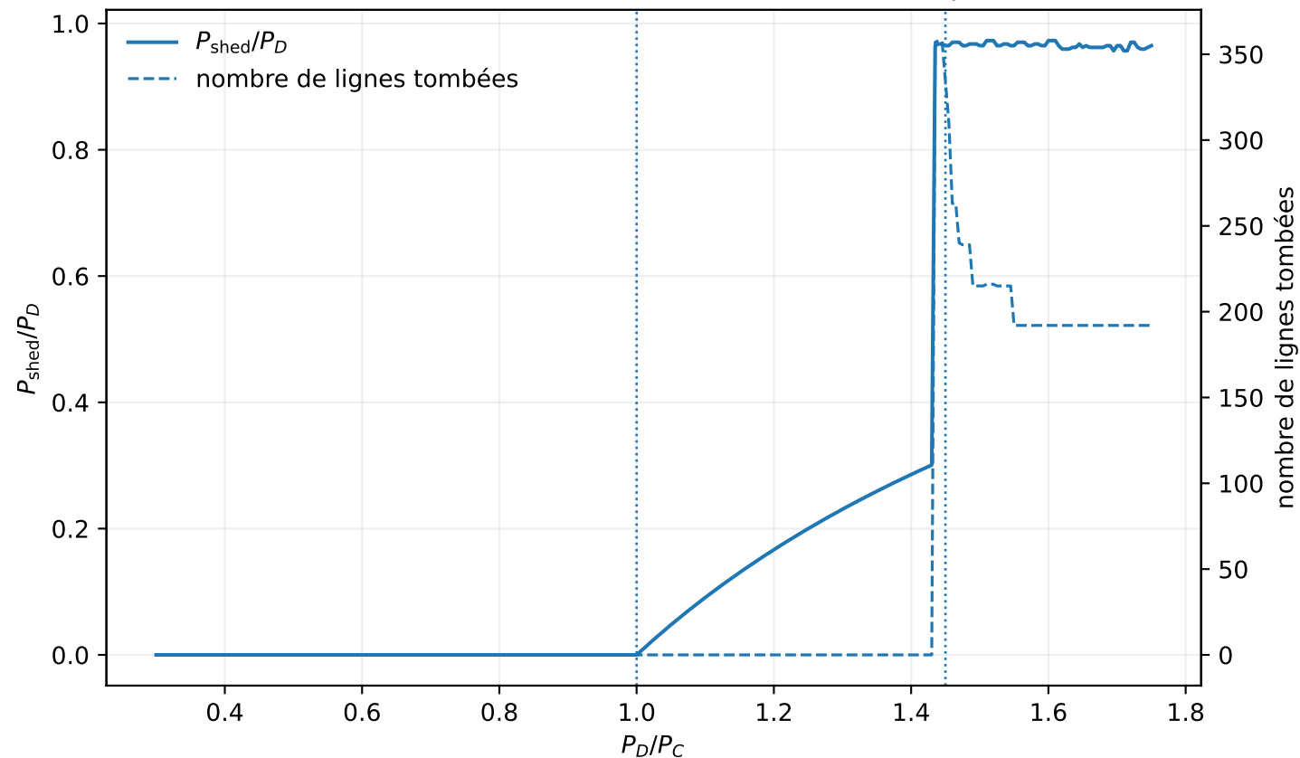
Transitions déterministes — arbre 382 nœuds, p_1 = 1
