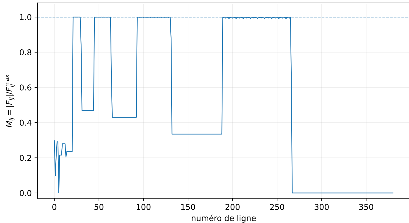
Lignes au voisinage de la limite de transport — P_D/P_C = 1.450 (initial)
