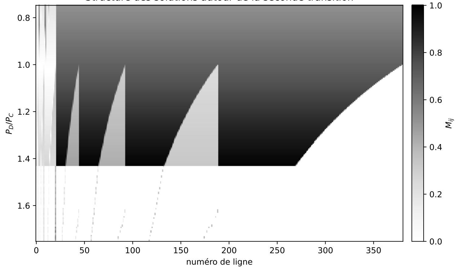
Structure des solutions autour de la seconde transition
