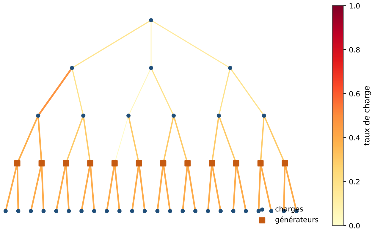
Taux de charge du réseau de 46 nœuds à P_D/P_C = 0.80
