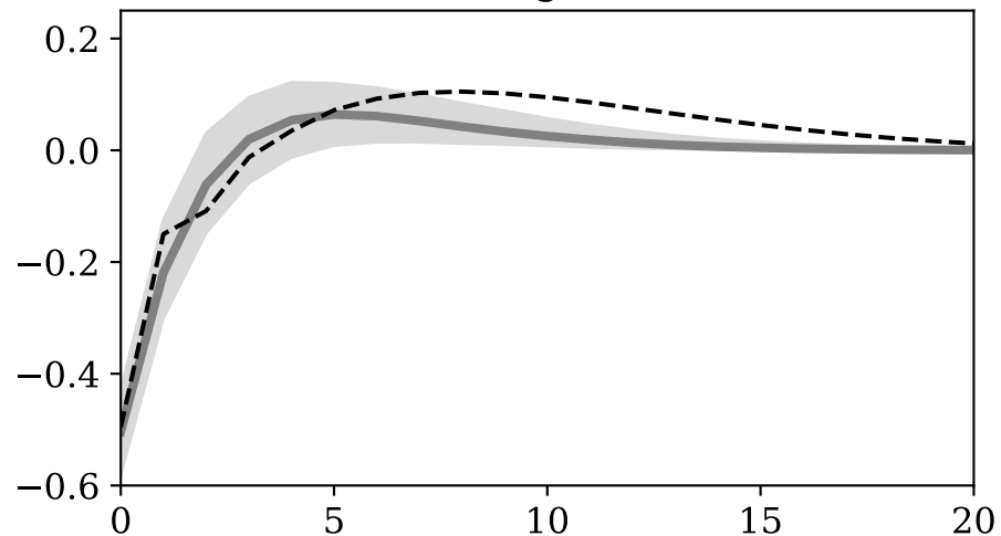
Vector autoregression (VAR)
