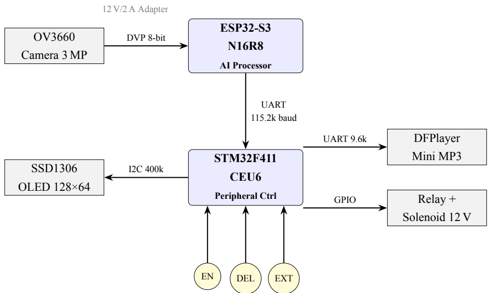
Hình A.1. Sơ đồ khối hệ thống STM-FaceGuard. Kiến trúc Dual-MCU: ESP32-S3 xử lý AI, STM32F411CEU6 điều khiển ngoại vi. Ba nút nhấn EN/DEL/EXT kết nối trực tiếp vào GPIO ngắt của STM32.
