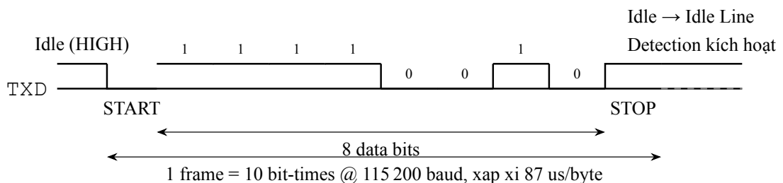
Hình A.2. UART Bit Timing Diagram (ví dụ byte 0 \times 4F = ký tự ‘O’). Idle Line Detection kích hoạt khi đường truyền giữ mức HIGH liên tục sau bit STOP, đánh dấu kết thúc một gói tin hoàn chỉnh.
