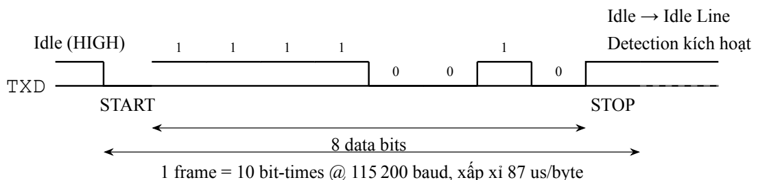
Hình A.2. UART Bit Timing Diagram (ví dụ byte 0x4F = ký tự ‘O’). Idle Line Detection kích hoạt khi đường truyền giữ mức HIGH liên tục sau bit STOP, đánh dấu kết thúc một gói tin hoàn chỉnh.
