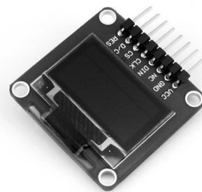
(b) Màn hình OLED SSD1306 0,96 inch tham chiếu.
