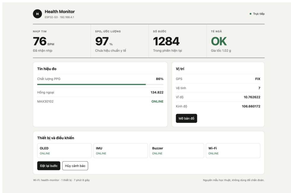
Figure 4: Dashboard web tinh gọn được render với dữ liệu minh họa để kiểm tra bố cục. Khi chạy trên ESP32-S3, trang lấy dữ liệu thực từ API JSON mỗi 0,25 giây.
