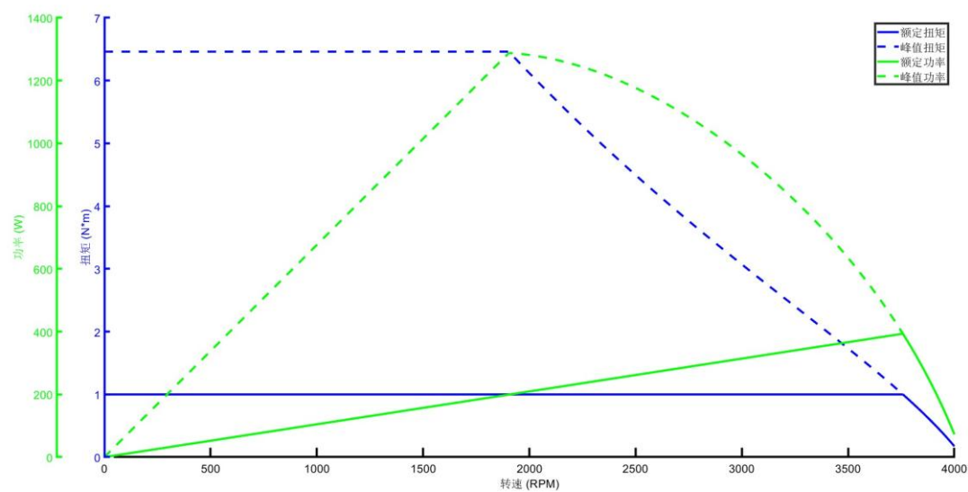
SEAF70A16NG01 关节电机外特性曲线
