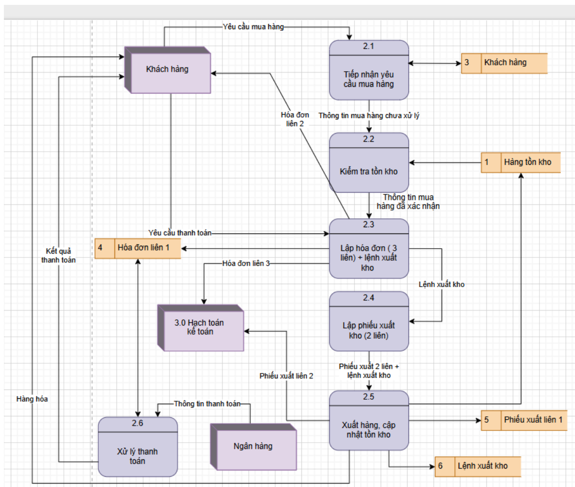
Hình 3.57: Mô hình DFD mức 2 của quy trình xử lý yêu cầu mua hàng
