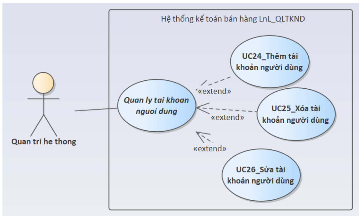
Hình 3.5: Sơ đồ use case mức chi tiết của quản lý tài khoản người dùng
