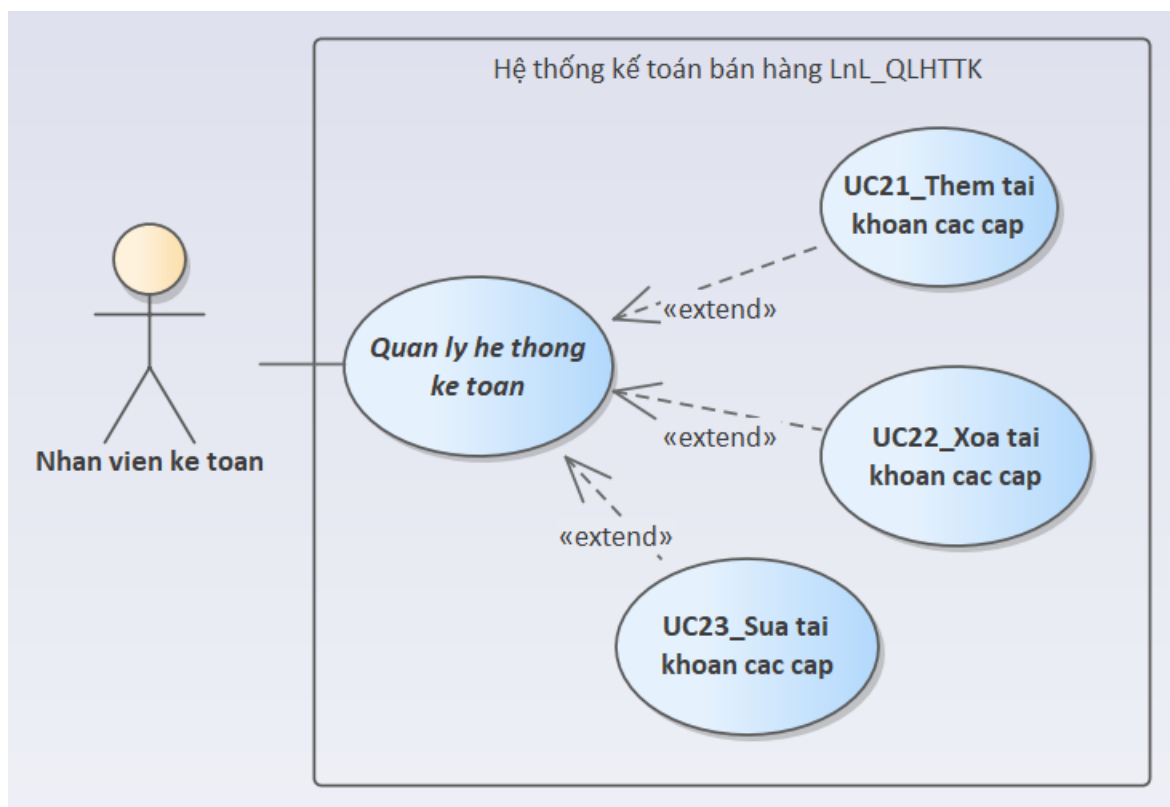
Hình 3.4: Sơ đồ use case mức chi tiết của quản lý hệ thống tài khoản
