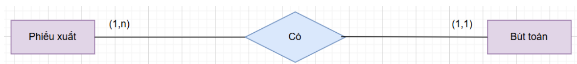
Hình 3.26: Mối quan hệ của Phiếu xuất và Bút toán
