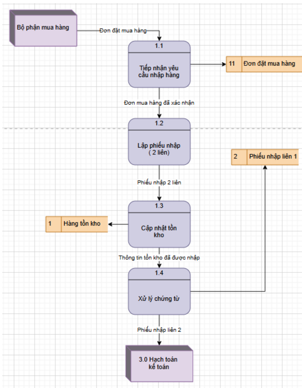
Hình 3.56: Mô hình DFD mức 2 của quy trình nhập hàng
