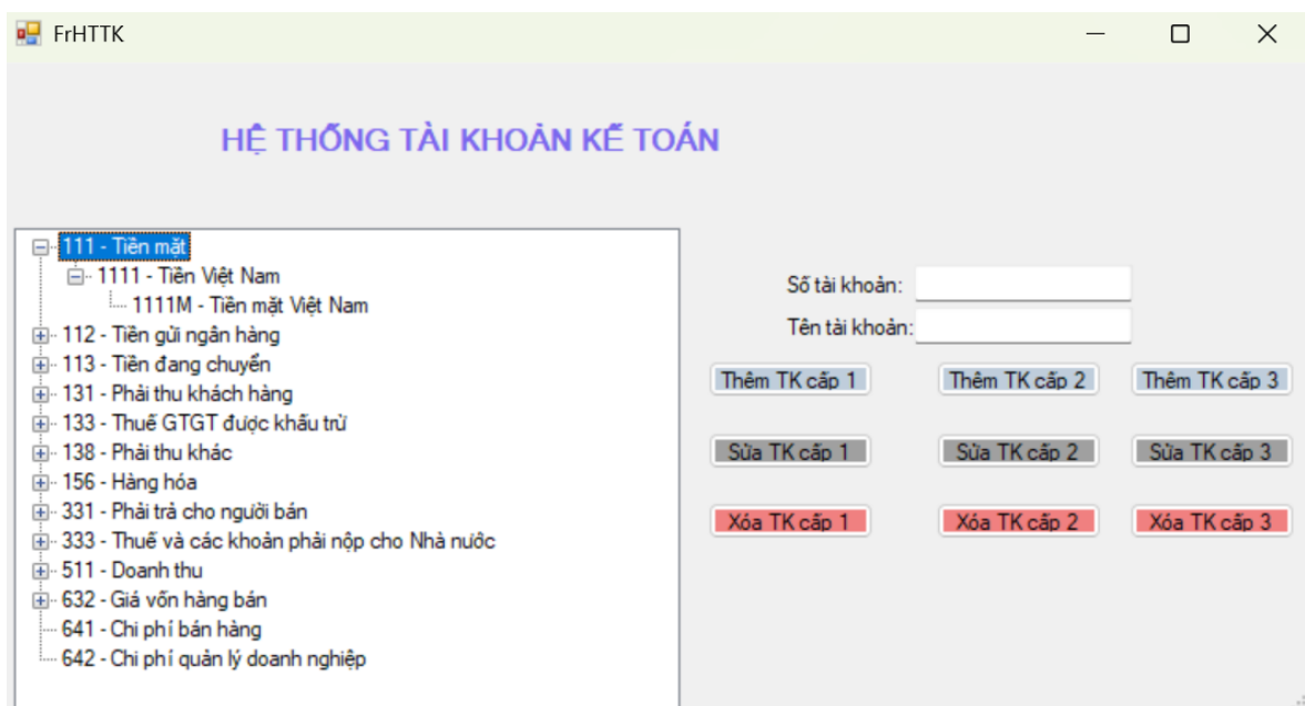
Hình 4.30: Màn hình quản lý hệ thống tài khoản kế toán
