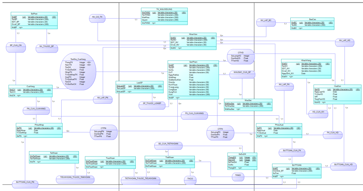
Hình 3.30: Mô hình dữ liệu mức quan niệm
