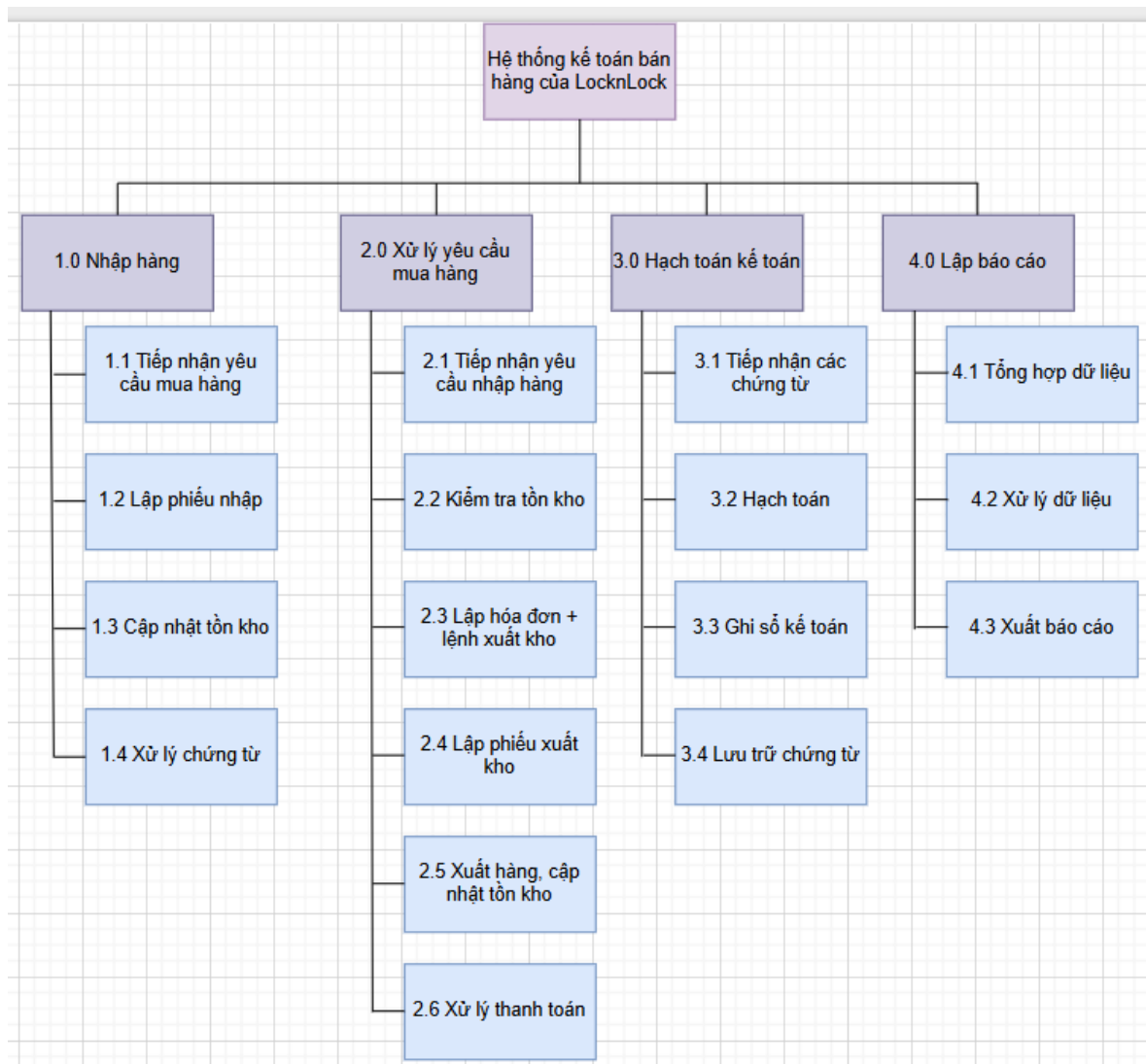
Hình 3.53: Mô hình BFD
