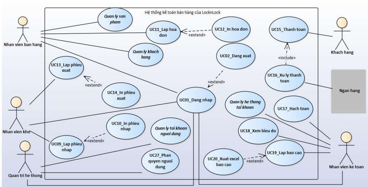
Hình 3.1: Sơ đồ use case mức tổng thể
