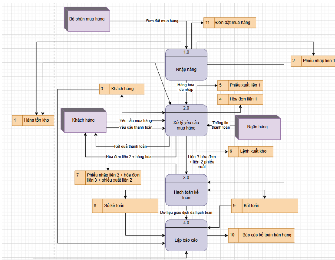
Hình 3.55: Mô hình DFD mức 1
