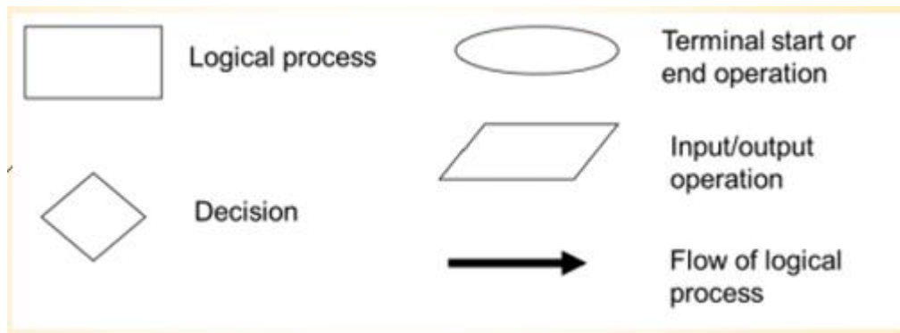
Hình 2.8: Bộ ký hiệu biểu diễn lưu đồ chương trình
