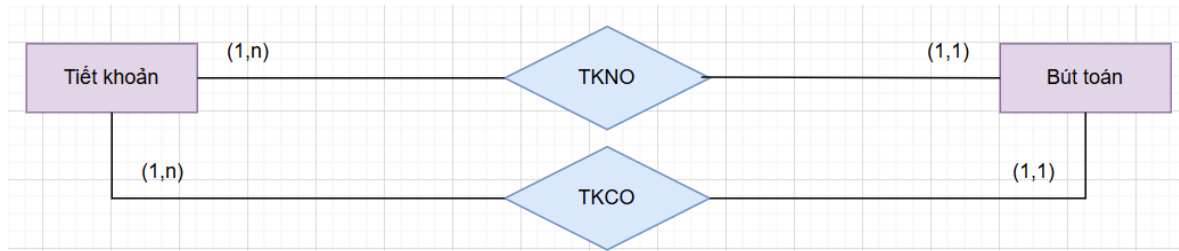
Hình 3.24: Mối quan hệ của Tiết khoản và Bút toán
