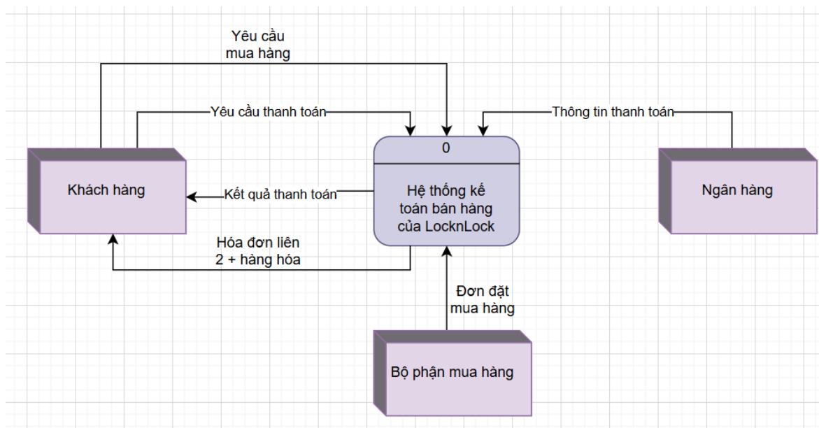
Hình 3.54: Mô hình DFD mức 0
