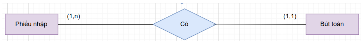
Hình 3.25: Mối quan hệ của Phiếu nhập và Bút toán
