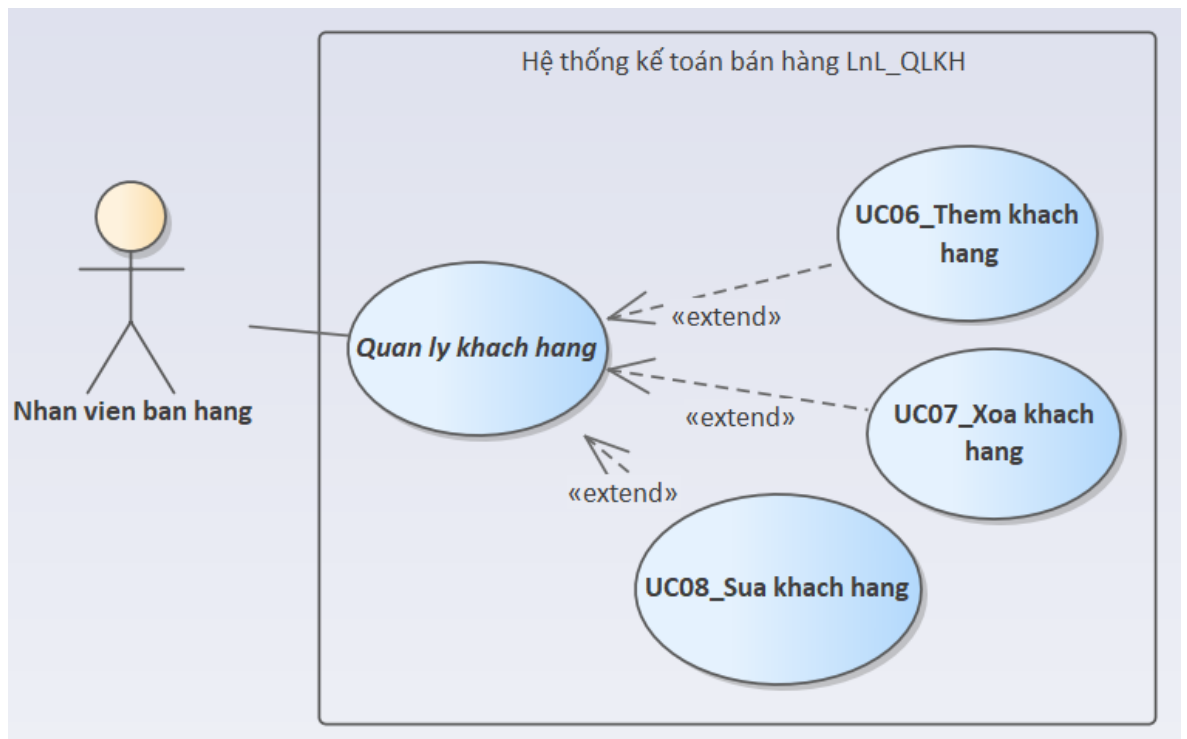
Hình 3.3: Sơ đồ use case mức chi tiết của quản lý khách hàng
