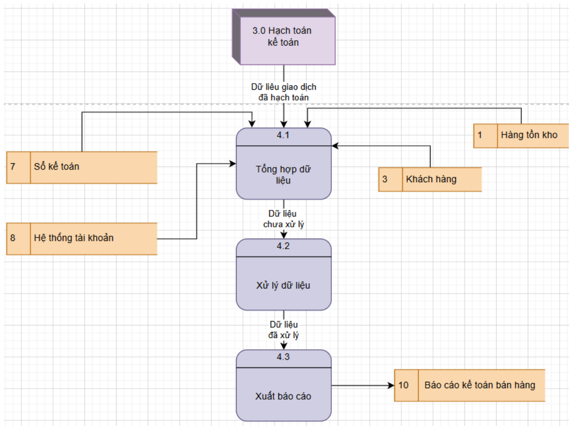
Hình 3.59: Mô hình DFD của quy trình Lập báo cáo
