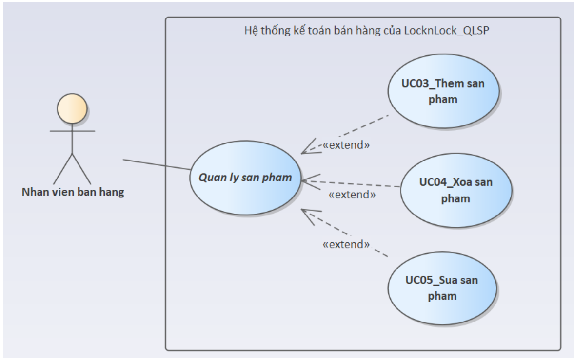
Hình 3.2: Sơ đồ use case mức chi tiết của quản lý sản phẩm
