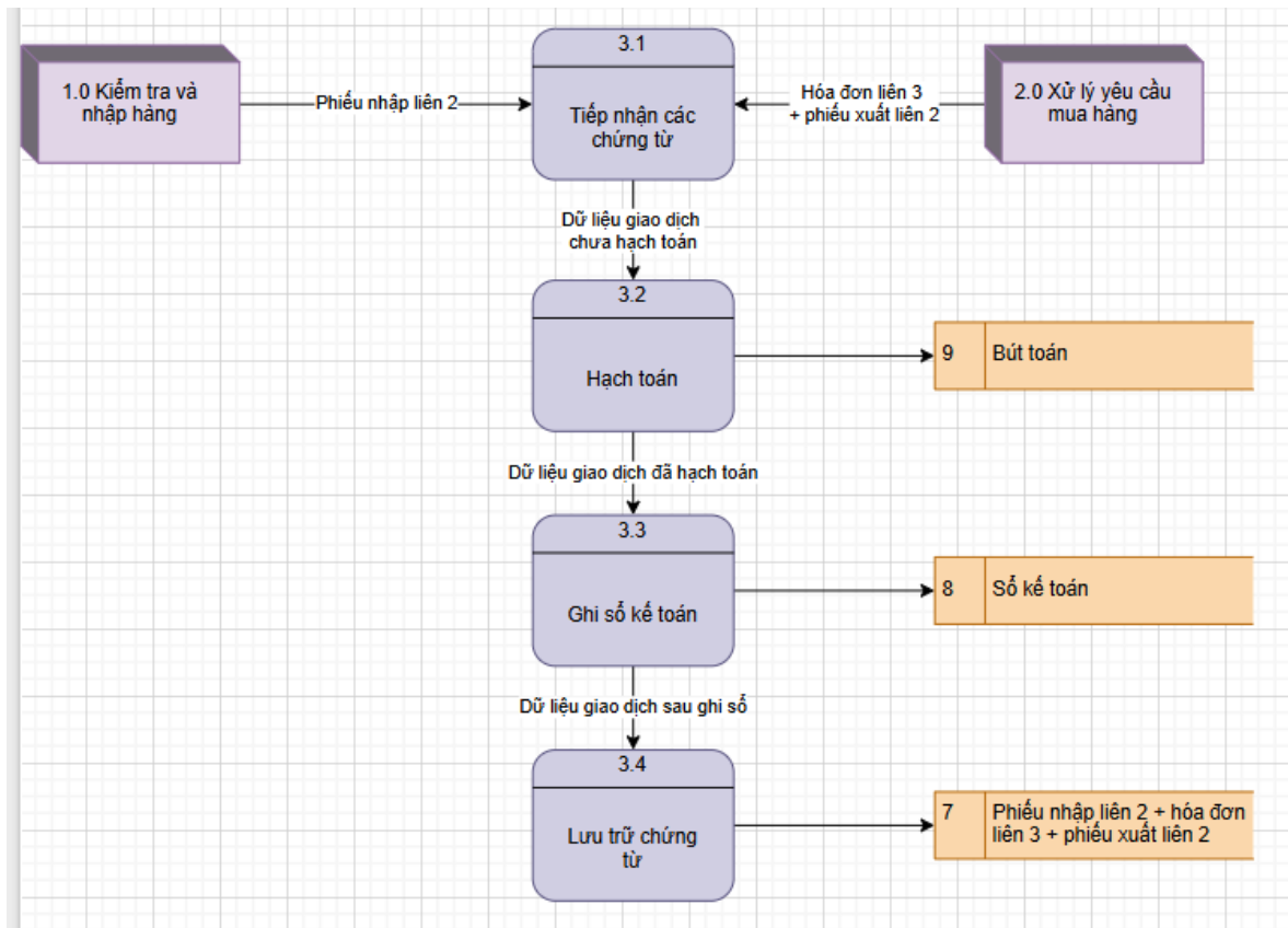
Hình 3.58: Mô hình DFD mức 2 của quy trình hạch toán kế toán
