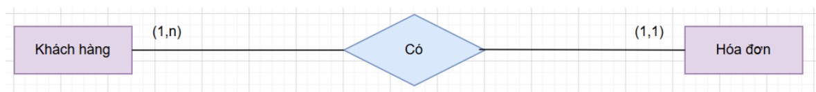
Hình 3.28: Mối quan hệ của Khách hàng và Hóa đơn
