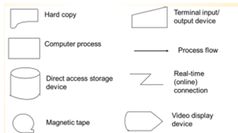
Hình 2.7: Bộ ký hiệu biểu diễn quy trình máy tính
