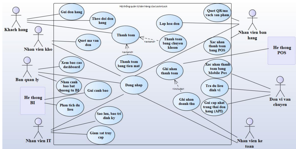
Hình 2.6: Sơ đồ Use case
