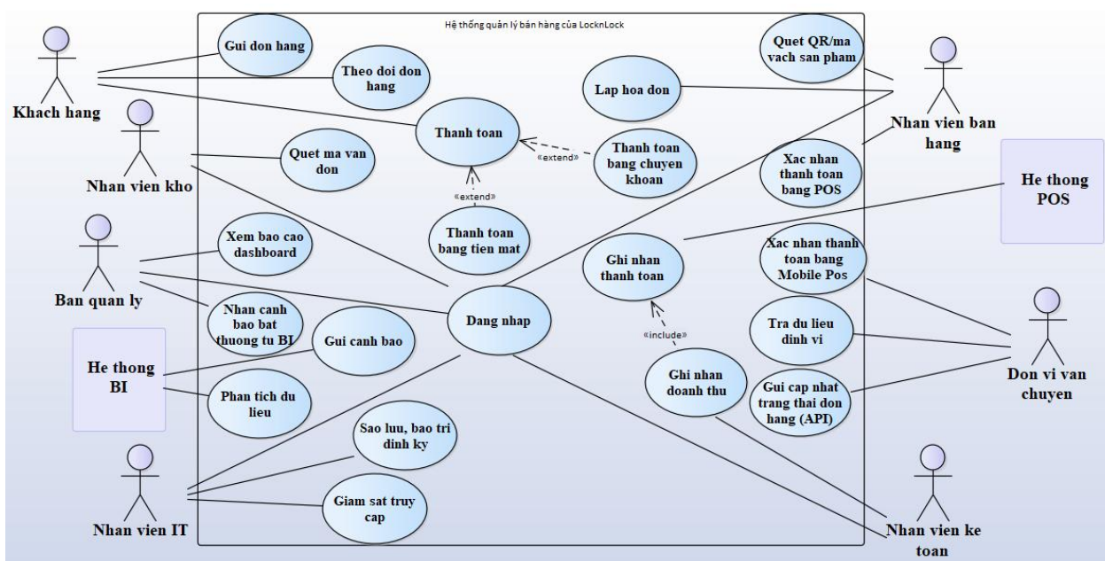
Hình 2.8: Sơ đồ Use case mô tả tác động giữa tác nhân và hệ thống
