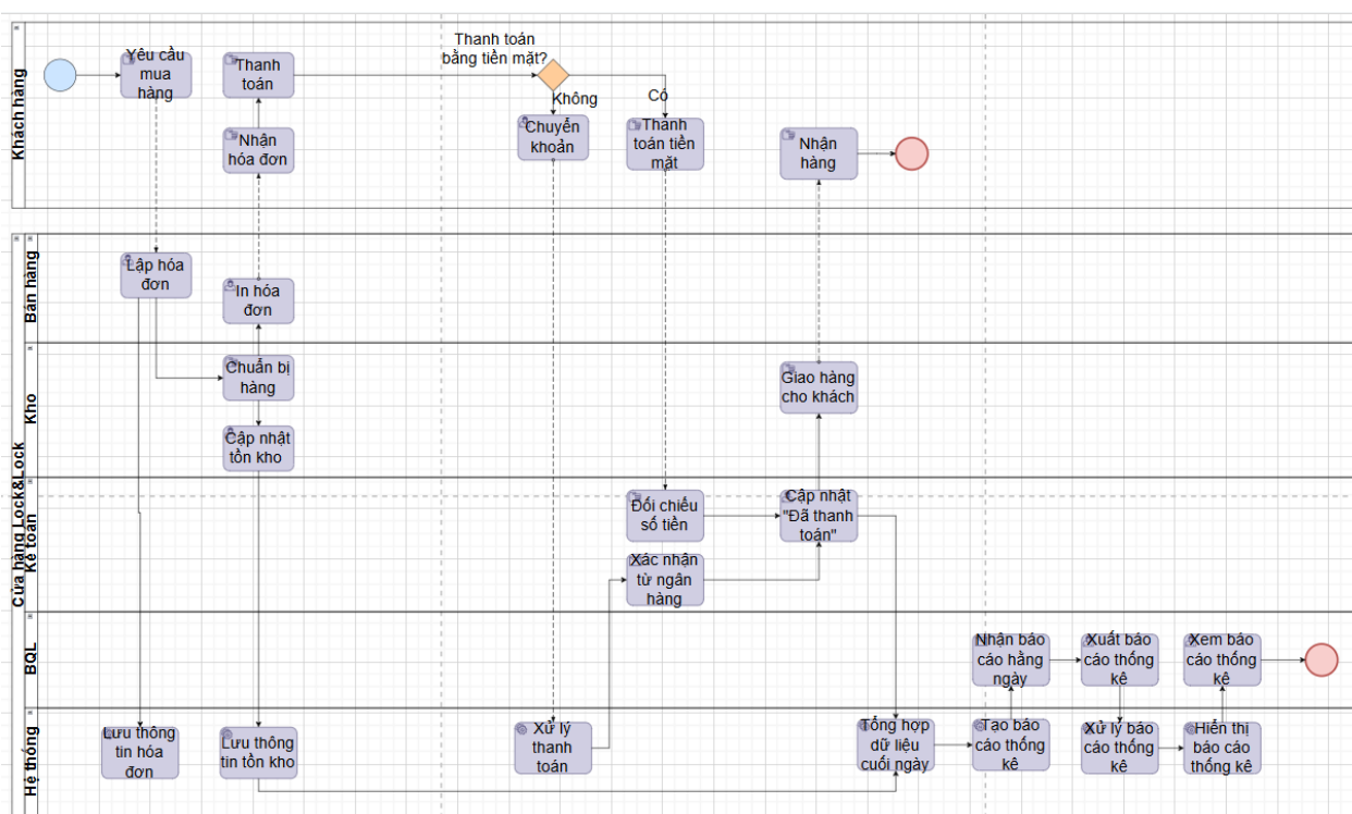
Hình 2.2: Mô hình BPMN cho quy trình offline
