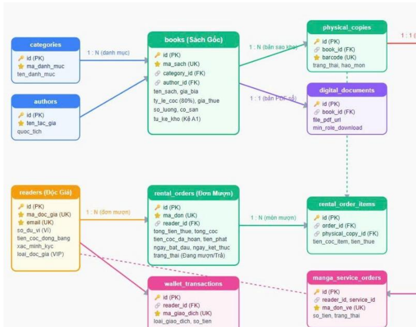
Hình 2.1: Sơ đồ Quan hệ Thực thể ERD Database (16+ Bảng)
