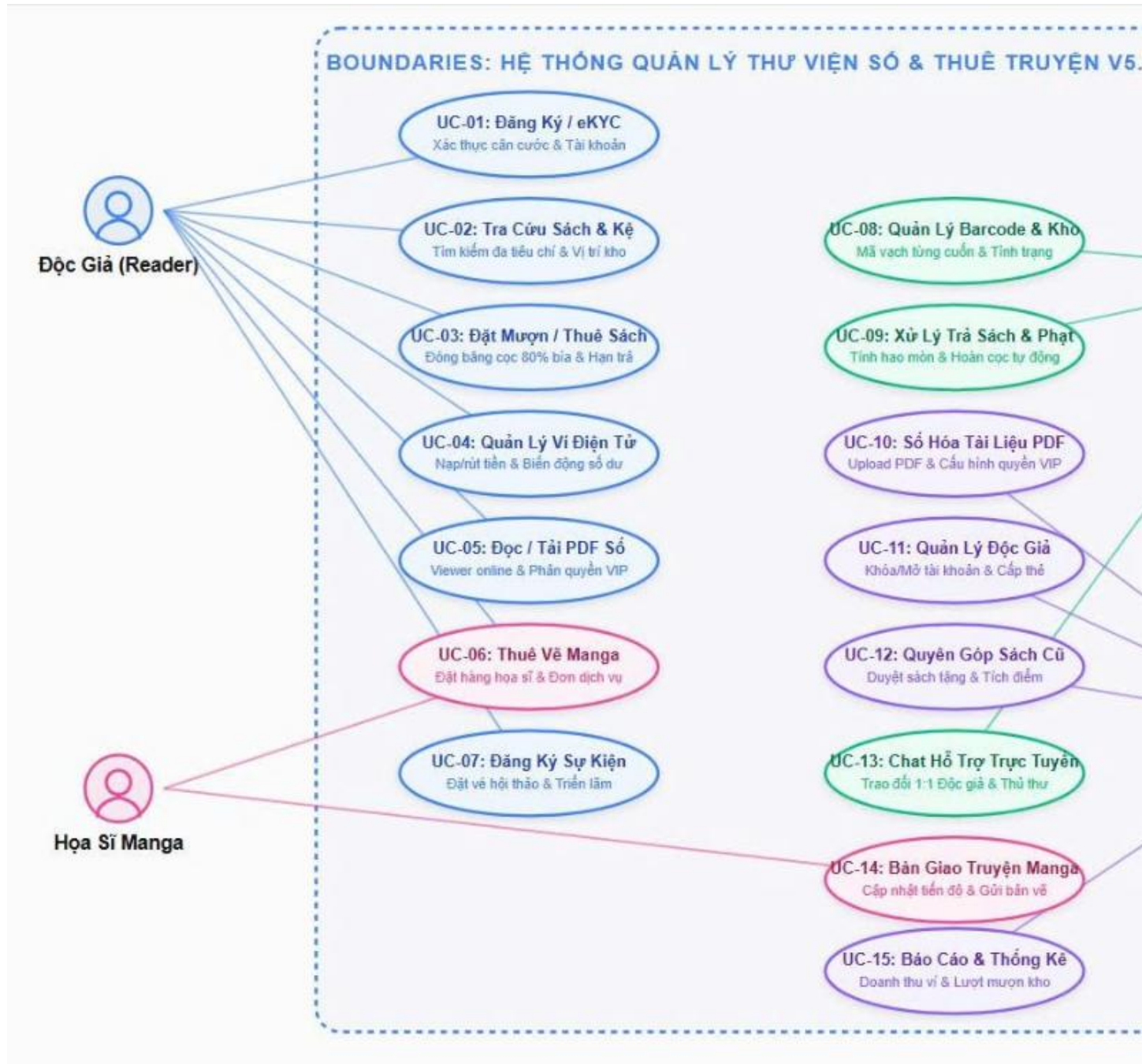
Hình 1.1: Sơ đồ Use Case Tổng Quan toàn hệ thống Enterprise v5.0
