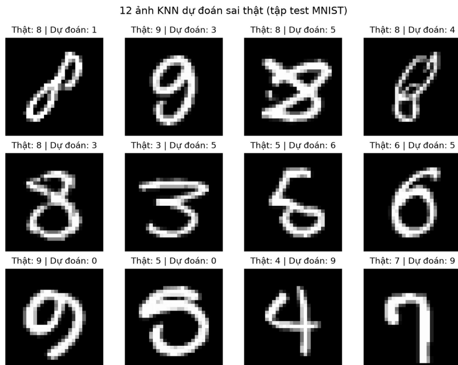
HÌNH 4.8: 12 ảnh KNN dự đoán sai thật, lấy ngẫu nhiên từ tập test
