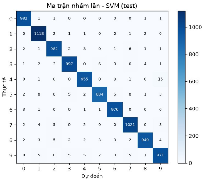
HÌNH 4.4: Ma trận nhầm lẫn của SVM trên tập test
