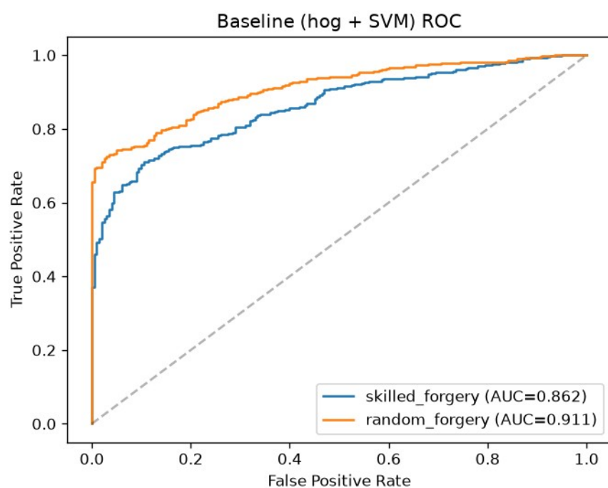
HÌNH 4.1: Đường cong ROC — baseline HOG + SVM (T1)
