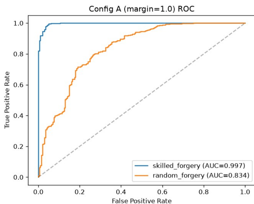
HÌNH 4.2: Đường cong ROC — Cấu hình A (T2)
