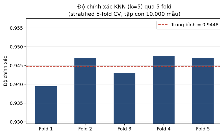
HÌNH 4.12: Biểu đồ độ chính xác KNN qua 5 fold
