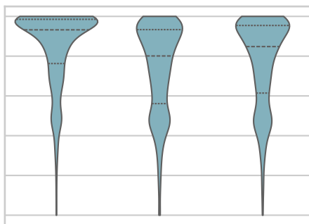
APIs
