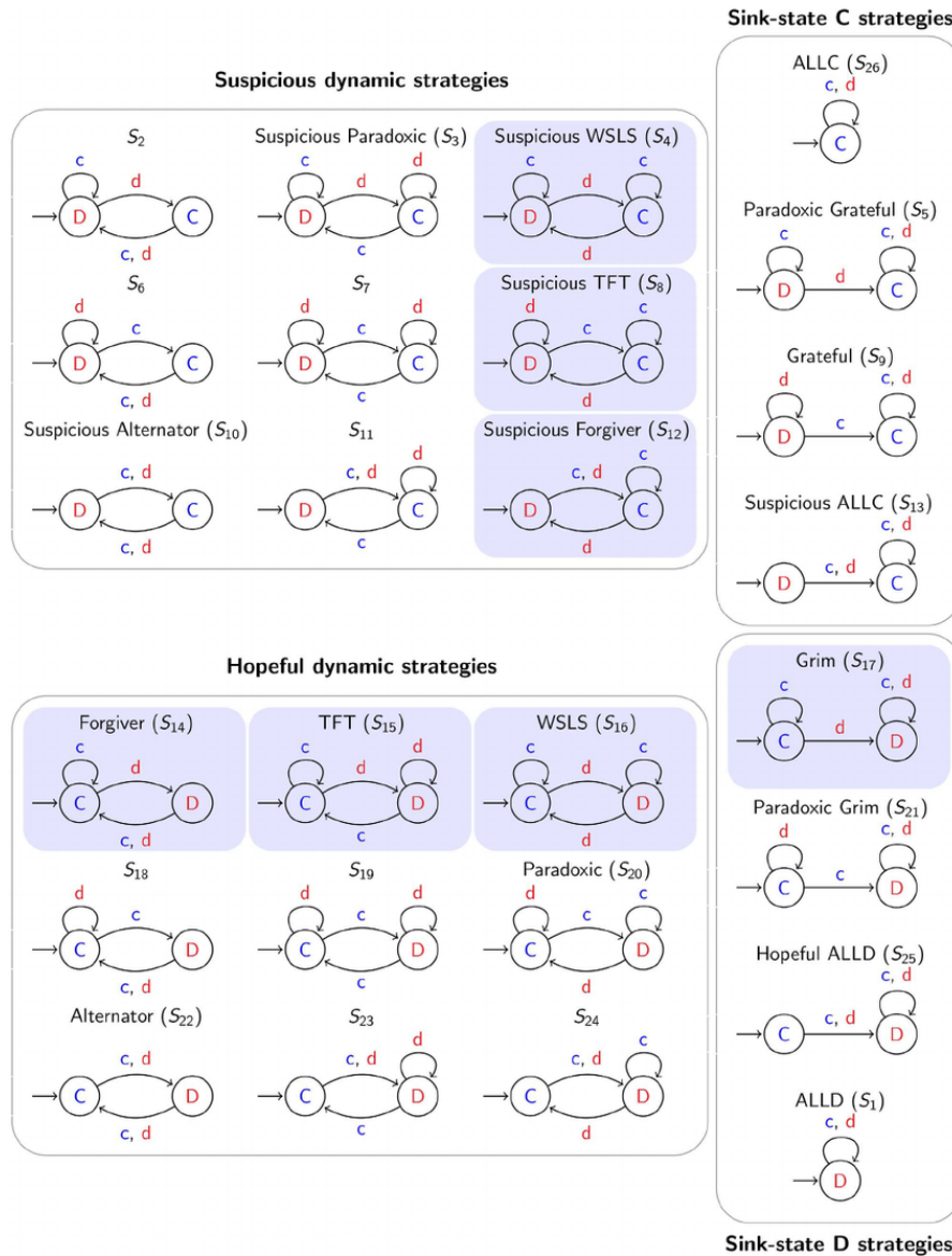
Gambar 3.1 Finite State Machine untuk strategi IPD oleh Reiter 2014
