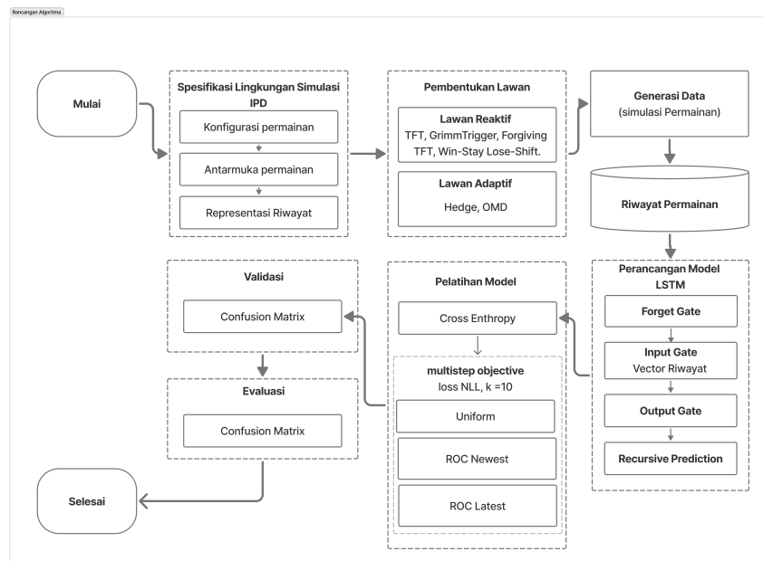
Gambar 4.2 Rancangan Algoritma Metode.
