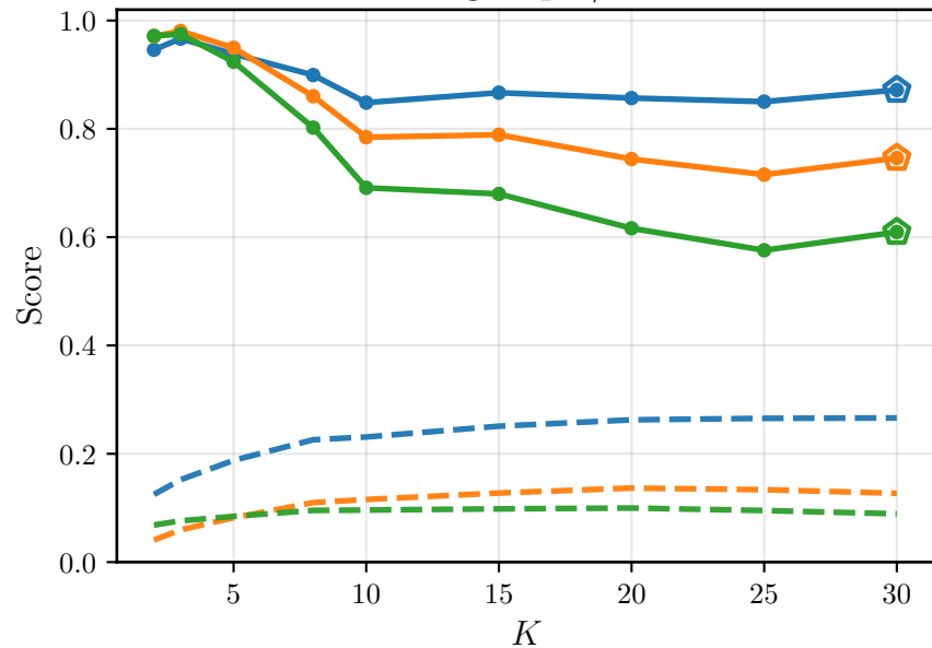
20 Newsgroups / t-SNE
