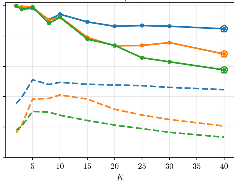
CIFAR-10 / UMAP
