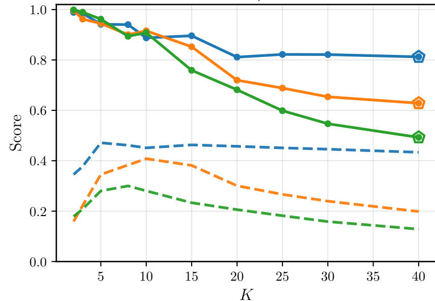
CIFAR-10 / t-SNE
