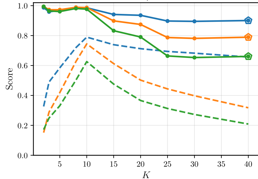
MNIST / t-SNE
