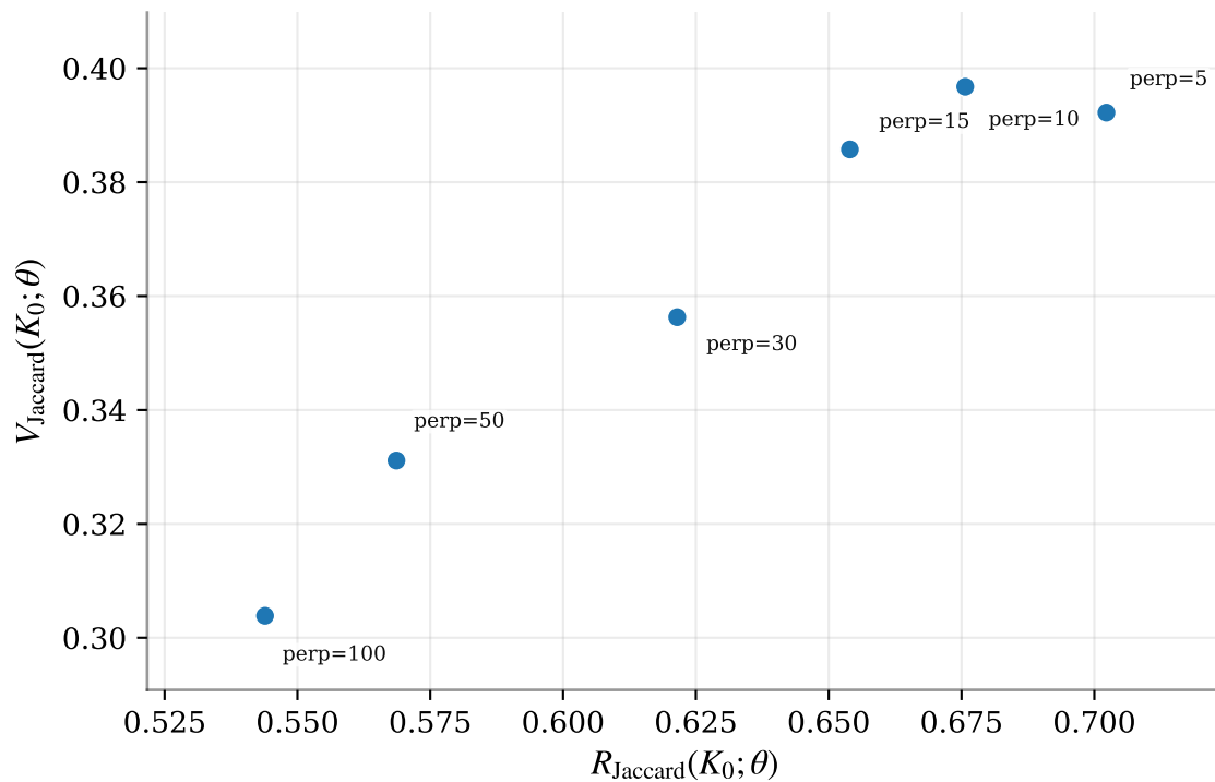
20 Newsgroups / t-SNE
