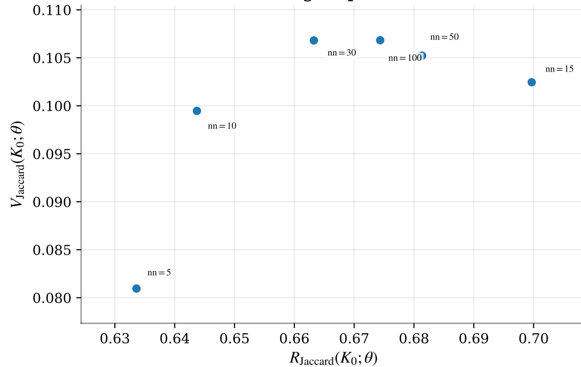
20 Newsgroups / UMAP
