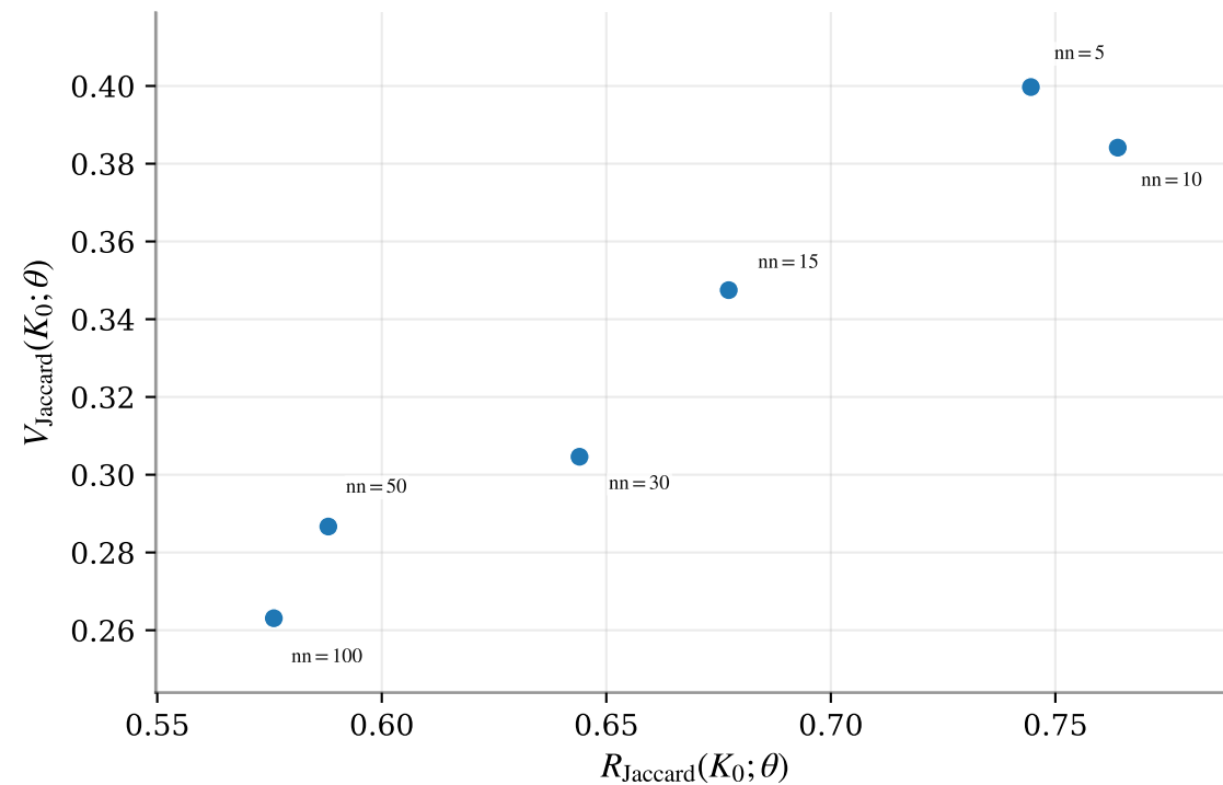
20 Newsgroups / UMAP
