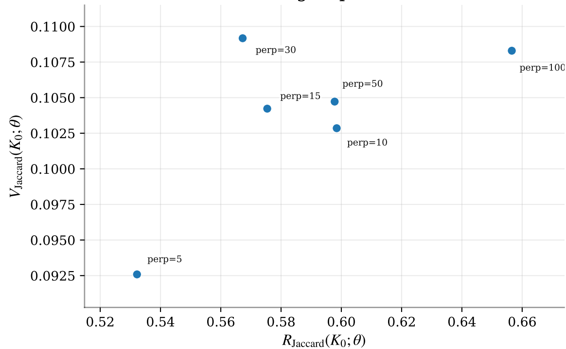
20 Newsgroups / t-SNE
