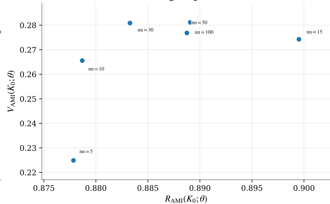
20 Newsgroups / UMAP
