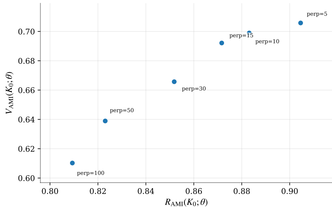
20 Newsgroups / t-SNE
