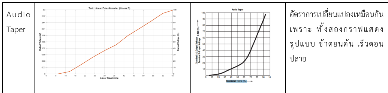
ตารางที่ 3 การเปรียบเทียบกราฟจากผลการทดลองกับกราฟจาก Datasheet
