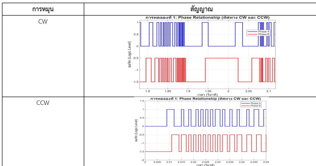
ตารางที่ 6 ความแตกต่างของสัญญาณเมื่อหมุน CW และ CCW
