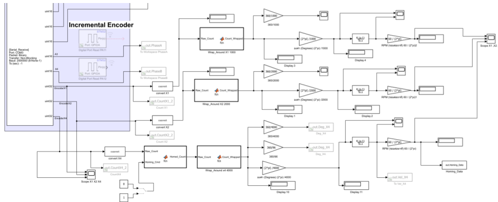
ภาพที่ 6 ภาพรวม Simulink ของ Encoder
