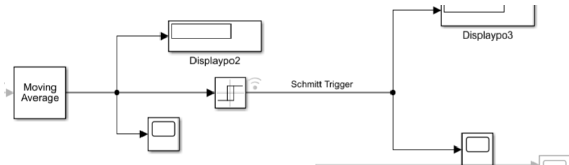
ภาพที่ 2 แปลงสัญญาณ Analog เป็น Digital
