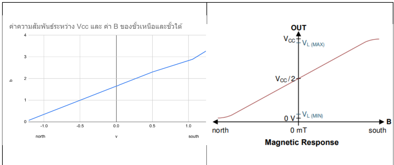
ตารางที่ 5 การเปรียบเทียบกราฟจากผลการทดลองกับ Datasheet
