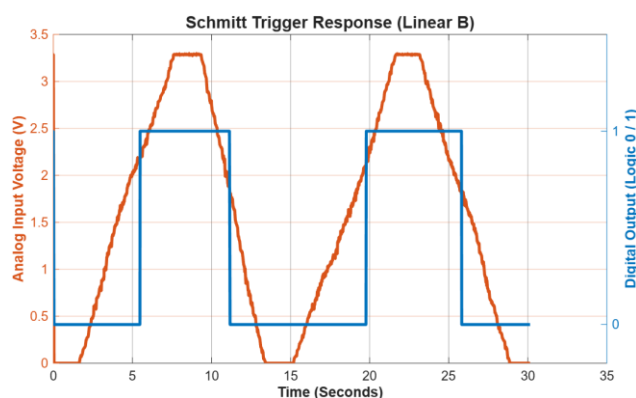
ภาพที่ 3 แปลงสัญญาณ Analog เป็น Digital
