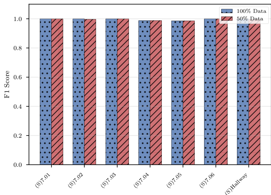
MLP
