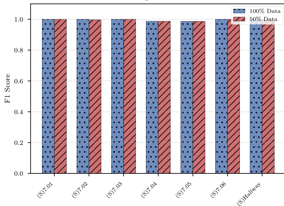
SVM
