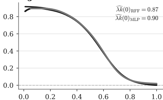
Sigmoidal BC
