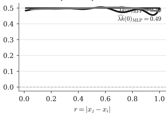
DeGroot (Linear)
