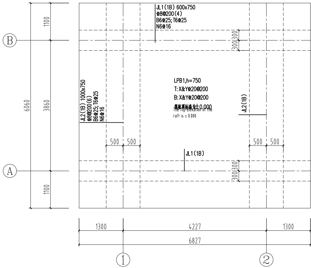
基础施工图
