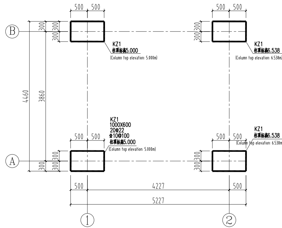
基础顶~6.538柱平法施工图
