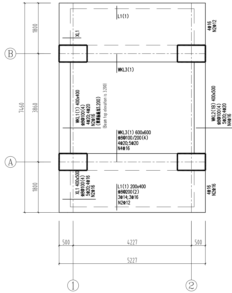
梁平法施工图
