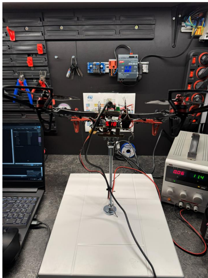
Rysunek 12: Stanowisko testowe
