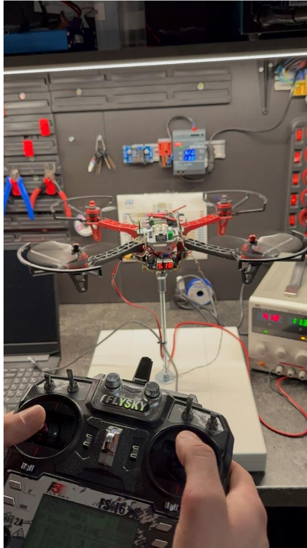
Rysunek 17: Dron podczas pozycji (0,0) w trakcie działania z poprawnie dobranymi parametrami PID
