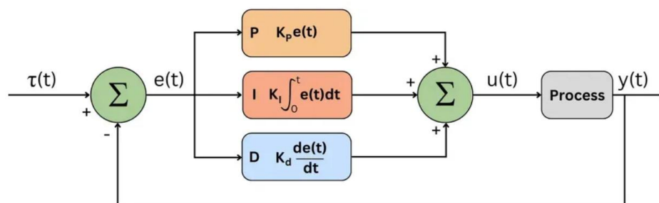
Rysunek 5: Schemat działania regulatora PID
