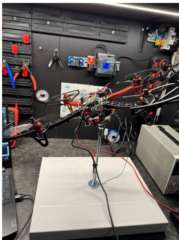
Rysunek 14: Testy Drona - start z pozycji maksymalnie wychylonej
