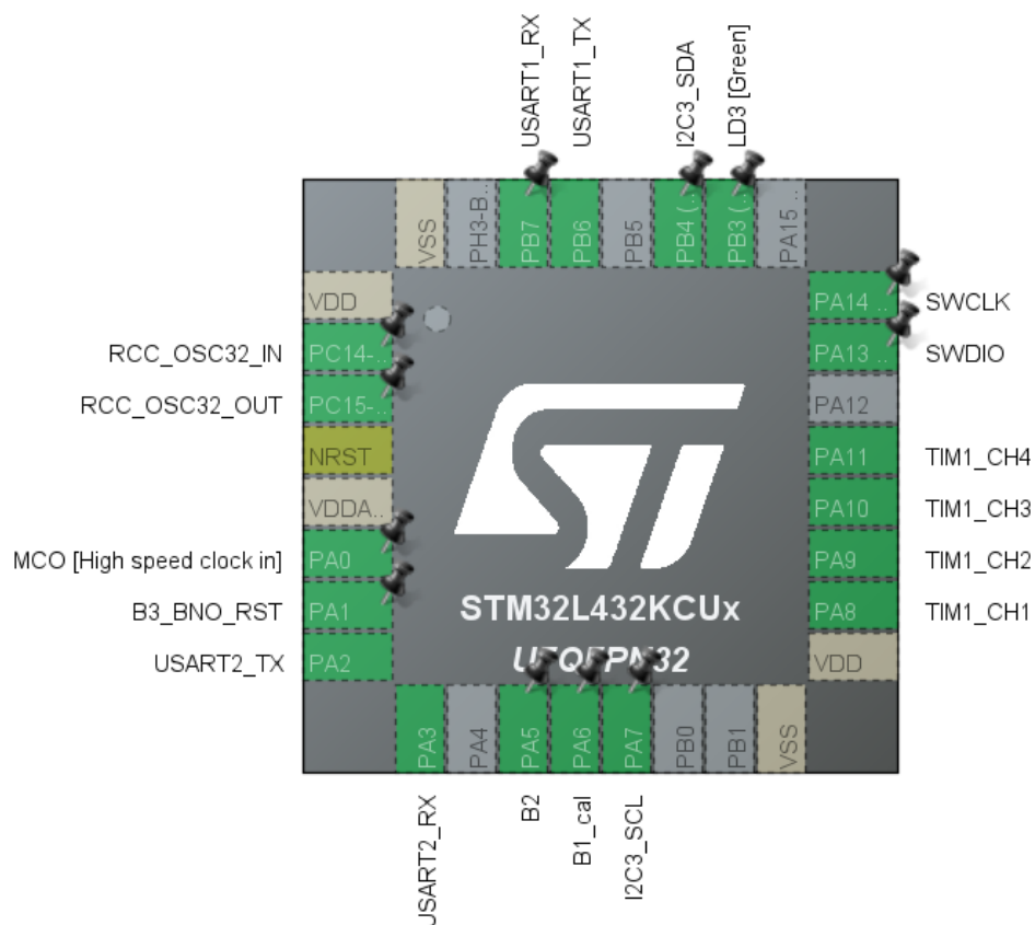
Rysunek 9: Konfiguracja Pinów mikrokontrolera STM32L432KC w programie STM32CubeMX
