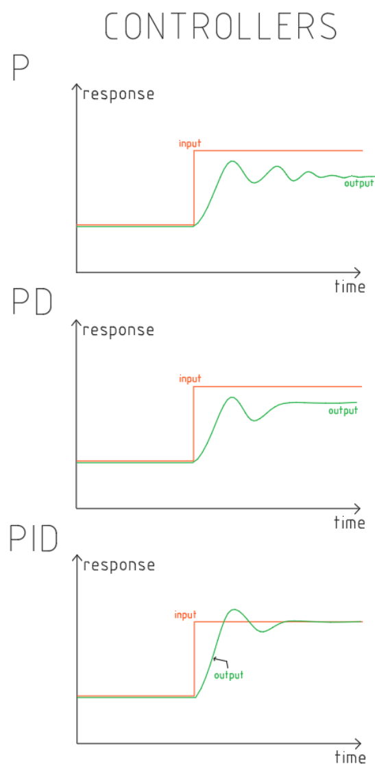
Rysunek 16: Wpływ poszczególnych członów regulatora PID na jego wyjście
