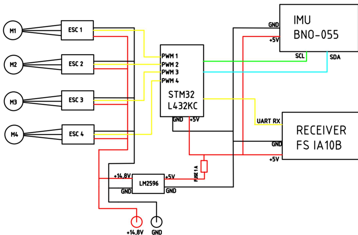
Rysunek 7: Diagram połączeń elektronicznych
