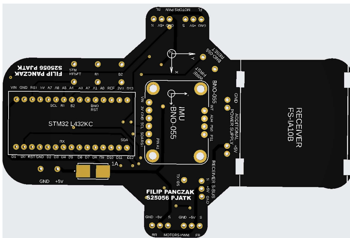
Rysunek 6: Dedykowana, autorska płytki PCB do sterowania dronem
