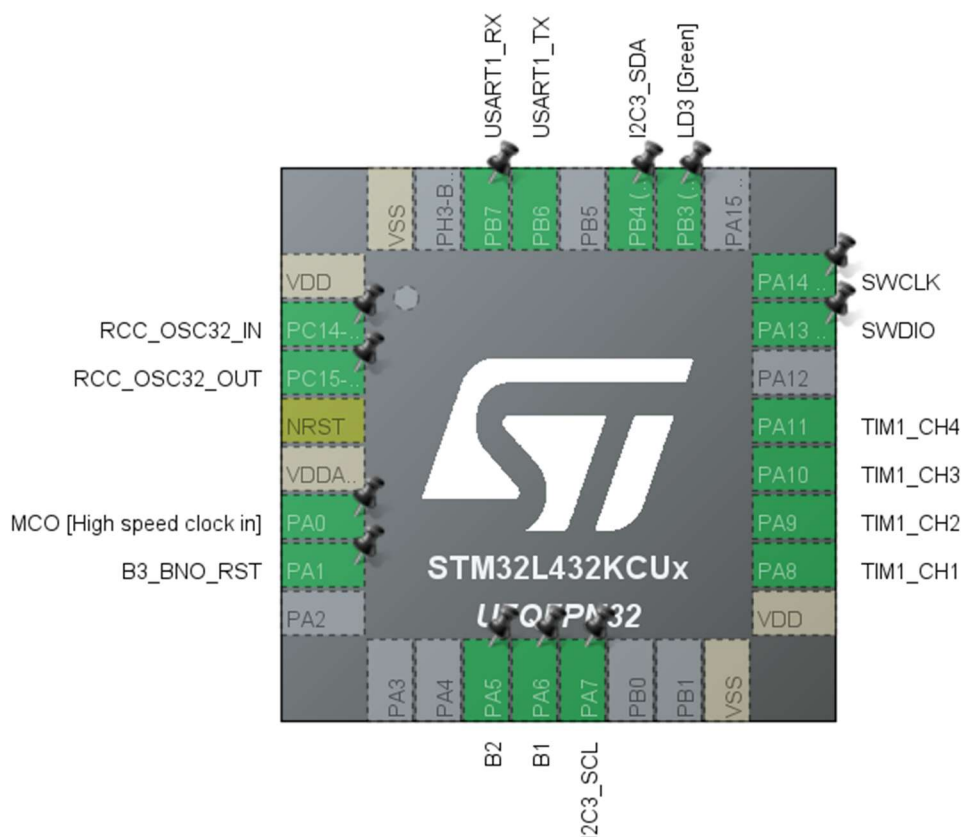
Rysunek 8: Konfiguracja Pinów mikrokontrolera STM32L432KC w programie STM32CubeMX
