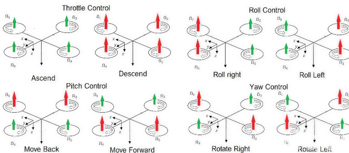
Rysunek 3: Wizualizacja sposobu kontroli osi Roll, Pitch, Yaw
