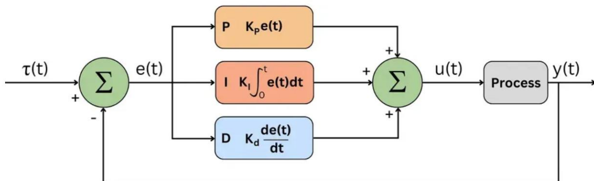
Rysunek 5: Schemat działania regulatora PID
