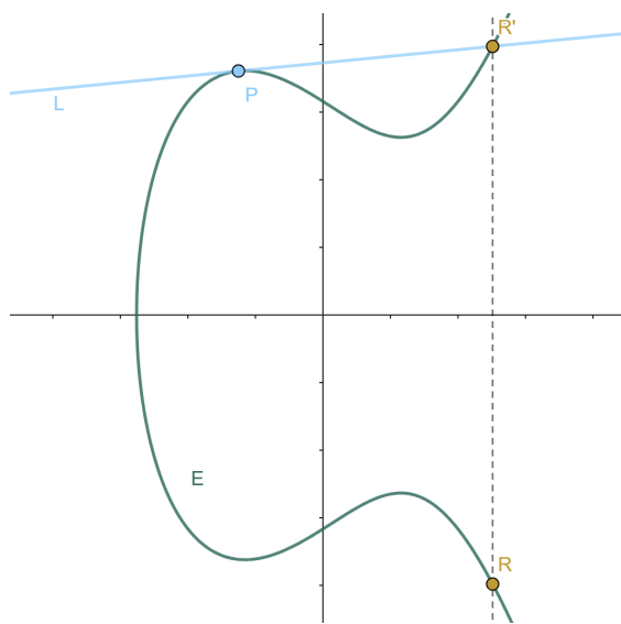
Abbildung 5. Spiegelung von R' und Konstruktion des Punktes R = 2P
