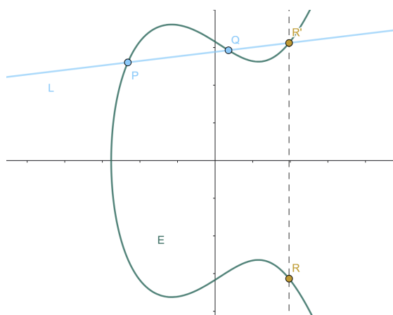
Abbildung 3. Dritter Schnittpunkt R' der Geraden L mit der Kurve E und Spiegelung an der x -Achse
