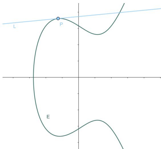
Abbildung 4. Tangente an die Kurve E im Punkt P
