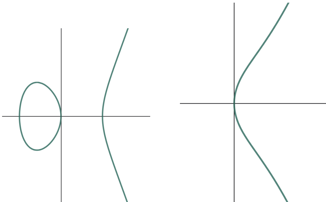
(a) Eigene Darstellung mit GeoGebra y^2 = x^3 - 3x
