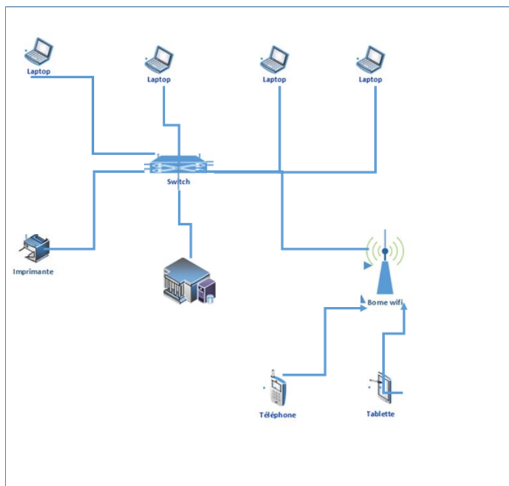
Figure 2 - Schéma de configuration du serveur national et infrastructure.
