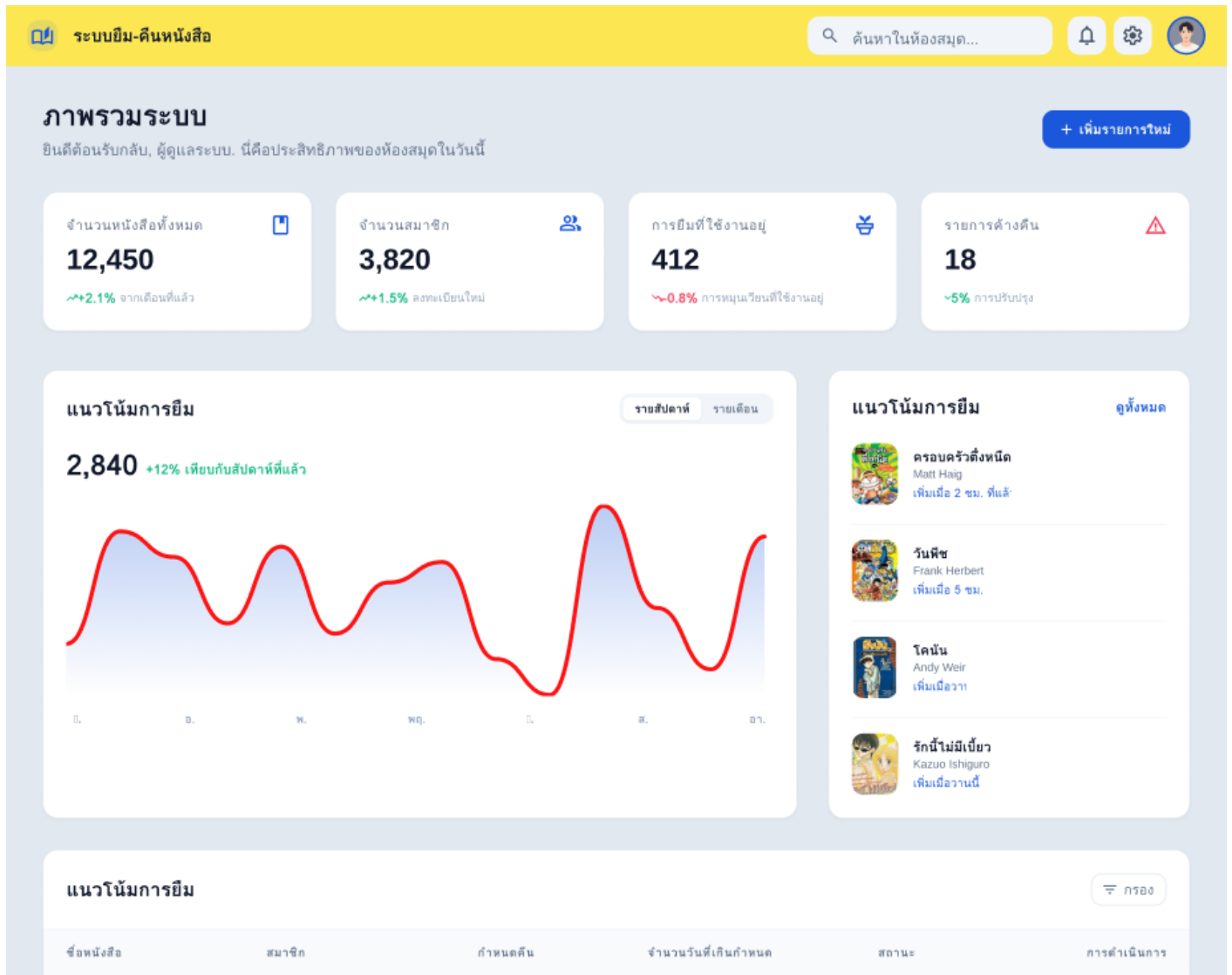
รูปที่ 7.6 หน้า UI ภาพรวมของระบบยืม-คืนหนังสือห้องสมุด
