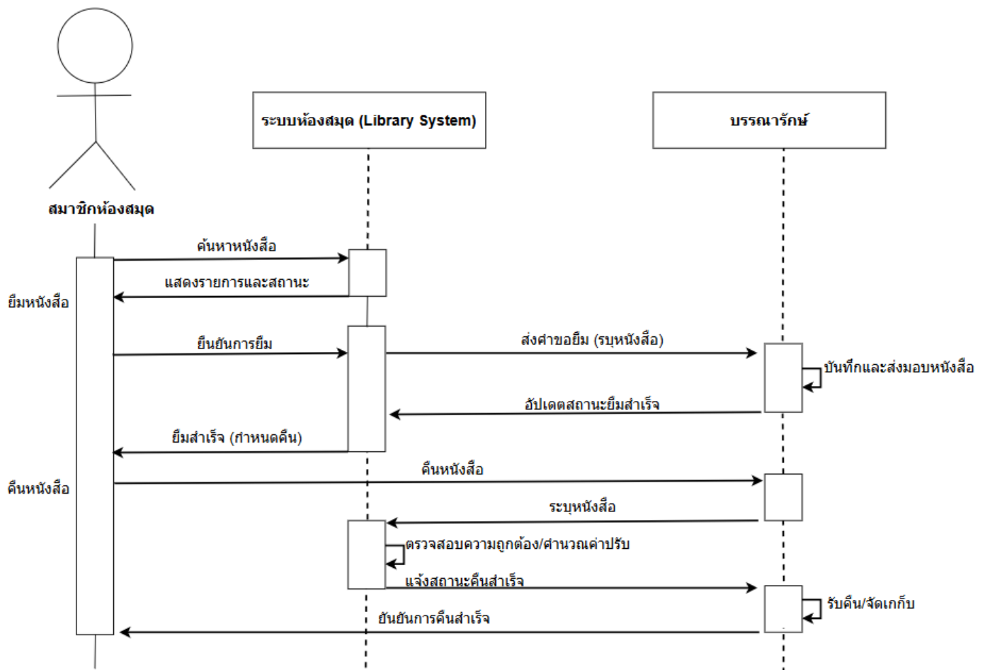
รูปที่ 8.4 Sequence Diagram ระบบยืม-คืนหนังสือ
