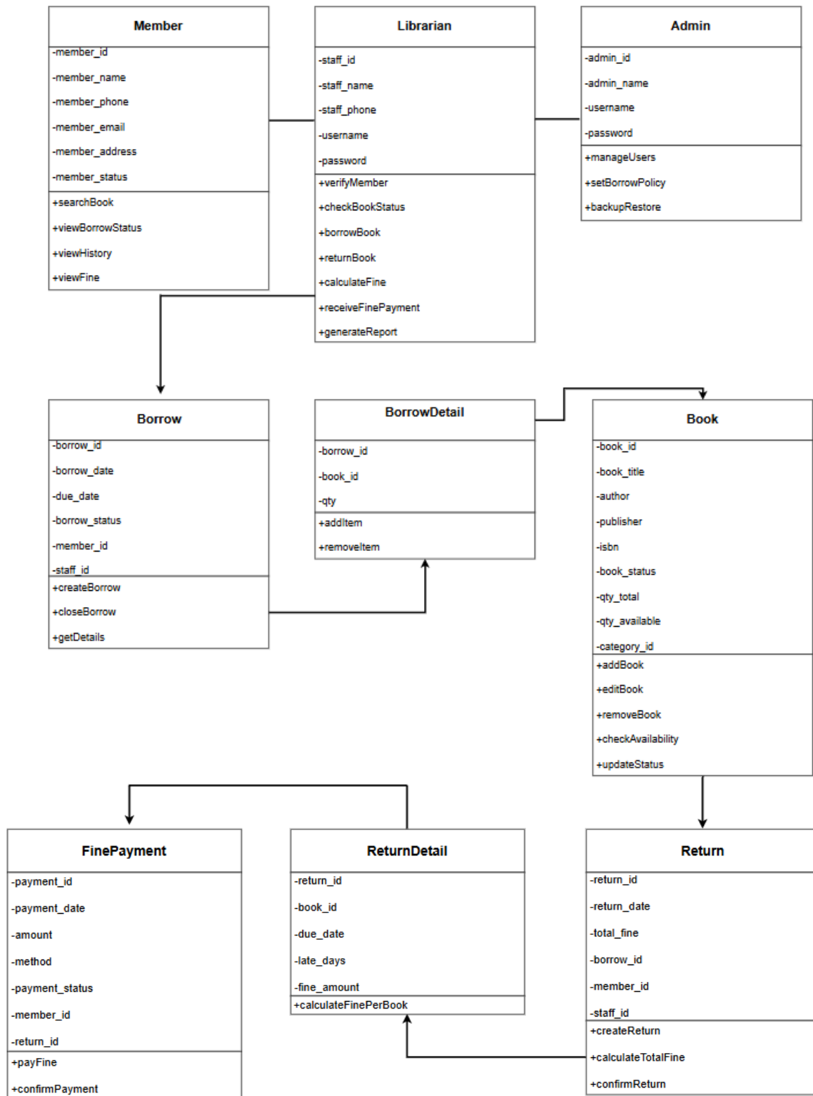
รูปที่ 8.2 Class Diagram
