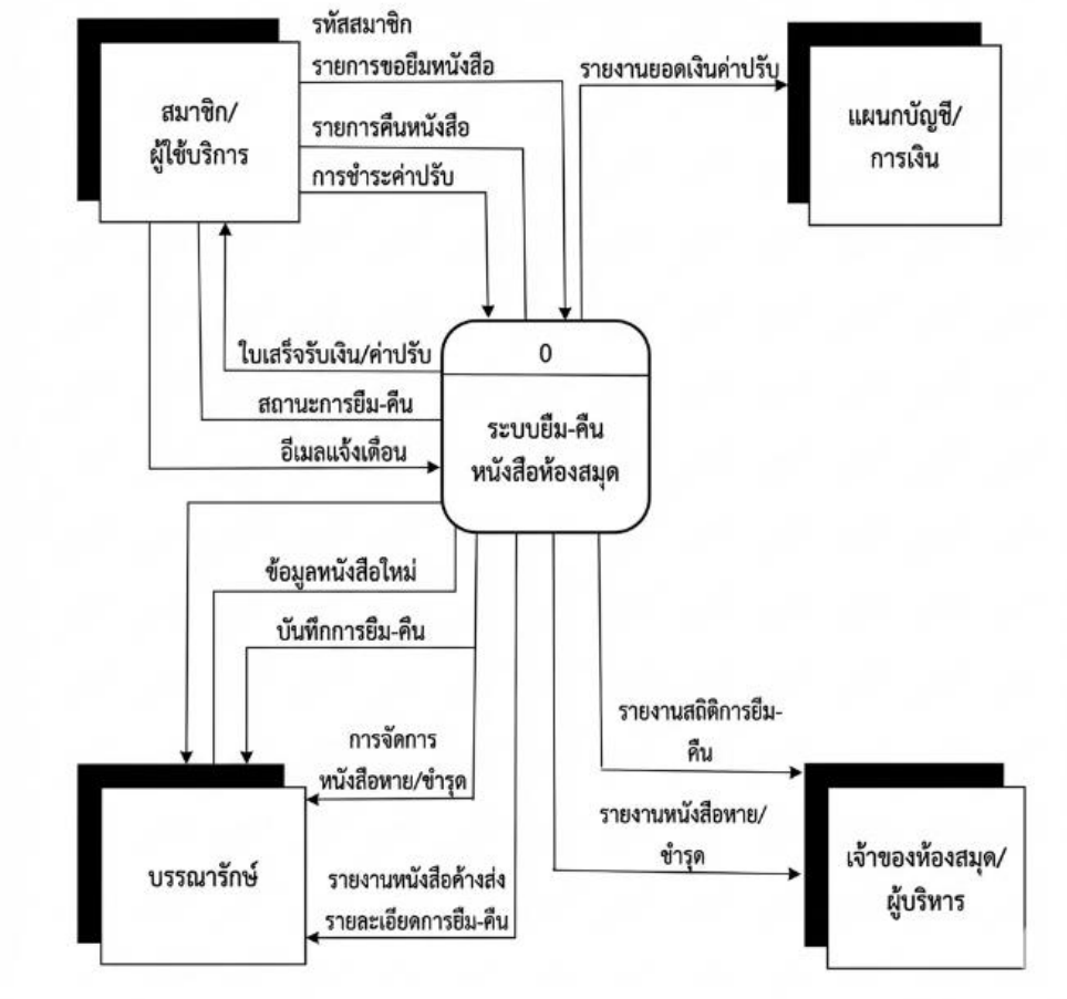
รูปที่ 2.2 Context Diagram ระบบยืม-คืนหนังสือห้องสมุด
