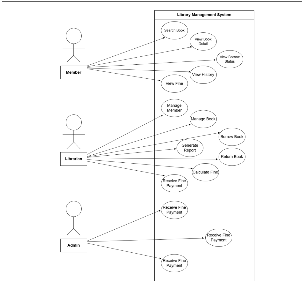
รูปที่ 8.1 Use-Case Diagrams
