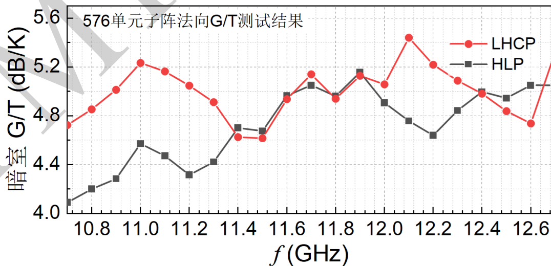
全频段法向波束 G/T 实测 (暗室数据)
