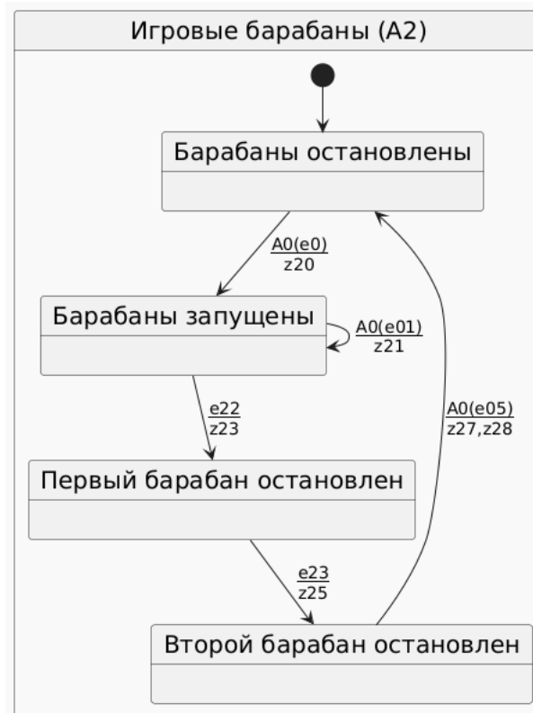
Рис. 3: Диаграмма состояний автомата A_2 (PlantUML, из puml/a2.puml ).
