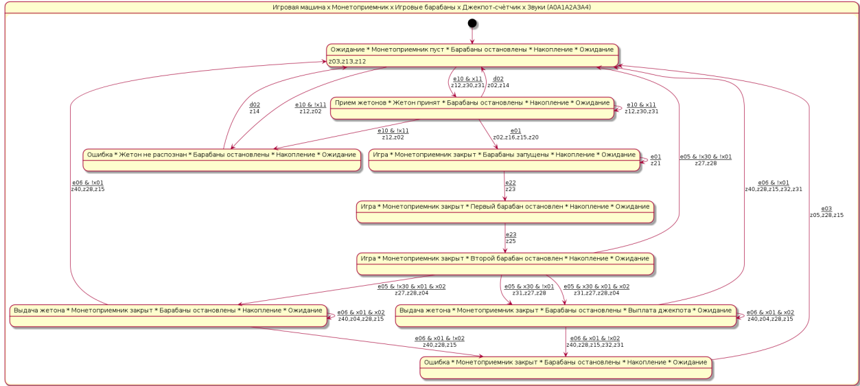
Рис. 6: Диаграмма состояний итогового автомата A_0 \times A_1 \times A_2 \times A_3 \times A_4 (PlantUML, из puml/final.puml ; 9 состояний).
