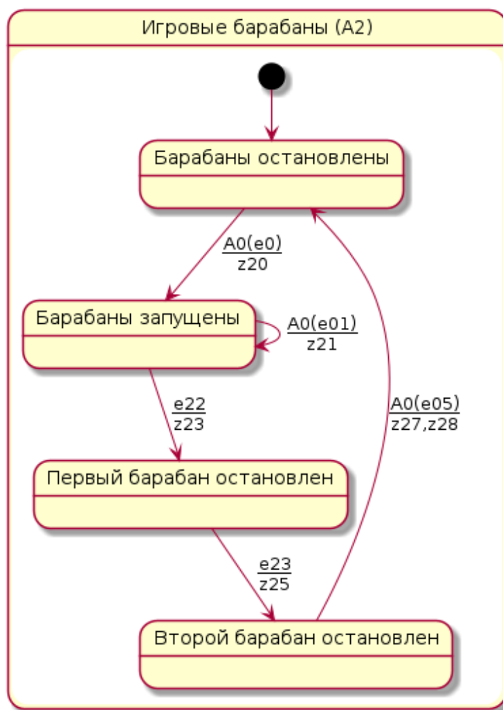
Рис. 3: Диаграмма состояний автомата A_2 (PlantUML, из puml/a2.puml ).
