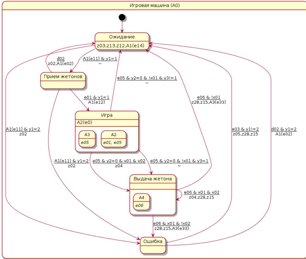
Рис. 1: Диаграмма состояний автомата A_0 (PlantUML, из puml/a0.puml ).
