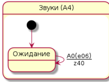
Рис. 5: Диаграмма состояний автомата A_4 (PlantUML, из puml/a4.puml ) — независимо вложенного автомата.
