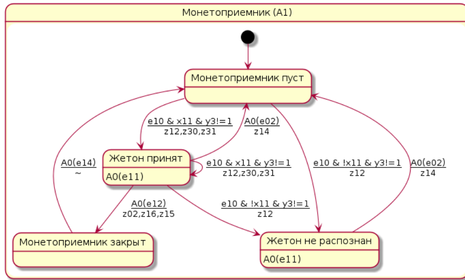
Рис. 2: Диаграмма состояний автомата A_1 (PlantUML, из puml/a1.puml ).
