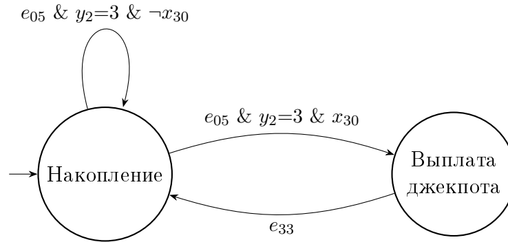
Рис. 4: Диаграмма состояний автомата A_3 — нового вложенного автомата.
