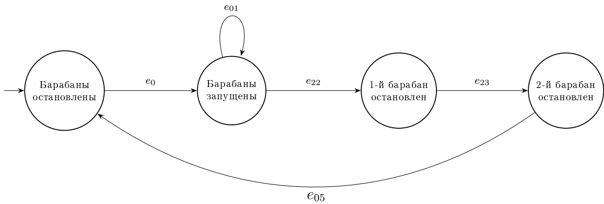
Рис. 3: Диаграмма состояний автомата A_2 .
