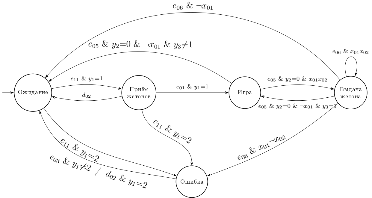
Рис. 1: Диаграмма состояний автомата A_0 .
