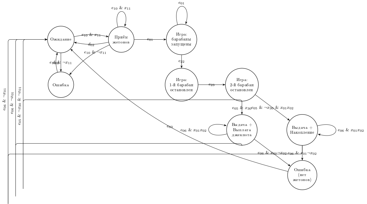
Рис. 5: Диаграмма состояний итогового автомата A_0 \times A_1 \times A_2 \times A_3 (9 состояний). Три длинных перехода сброса в «Ожидание» (из q_4, q_5, q_6 ) намеренно разведены по внешнему контуру, чтобы не пересекать основной поток диаграммы.
