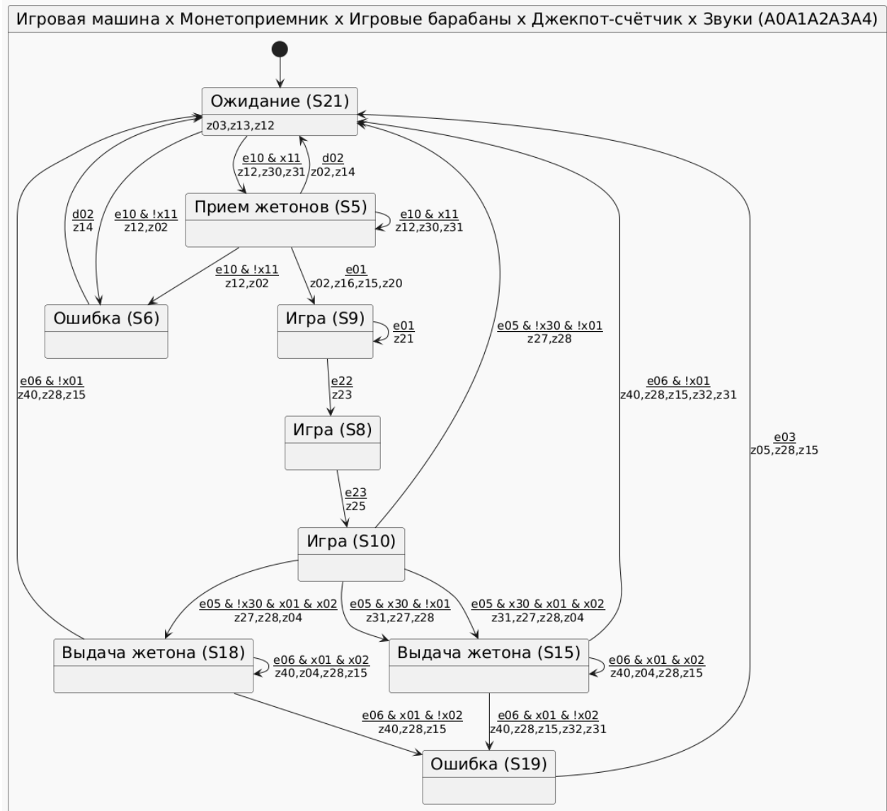
Рис. 6: Диаграмма состояний итогового автомата A_0 \times A_1 \times A_2 \times A_3 \times A_4 (PlantUML, из puml/final.puml ; 9 состояний). Каждое составное состояние подписано именем состояния A_0 (ведущего автомата) — полное соответствие номера состояния всем пяти исходным состояниям приведено в примечании ниже.
