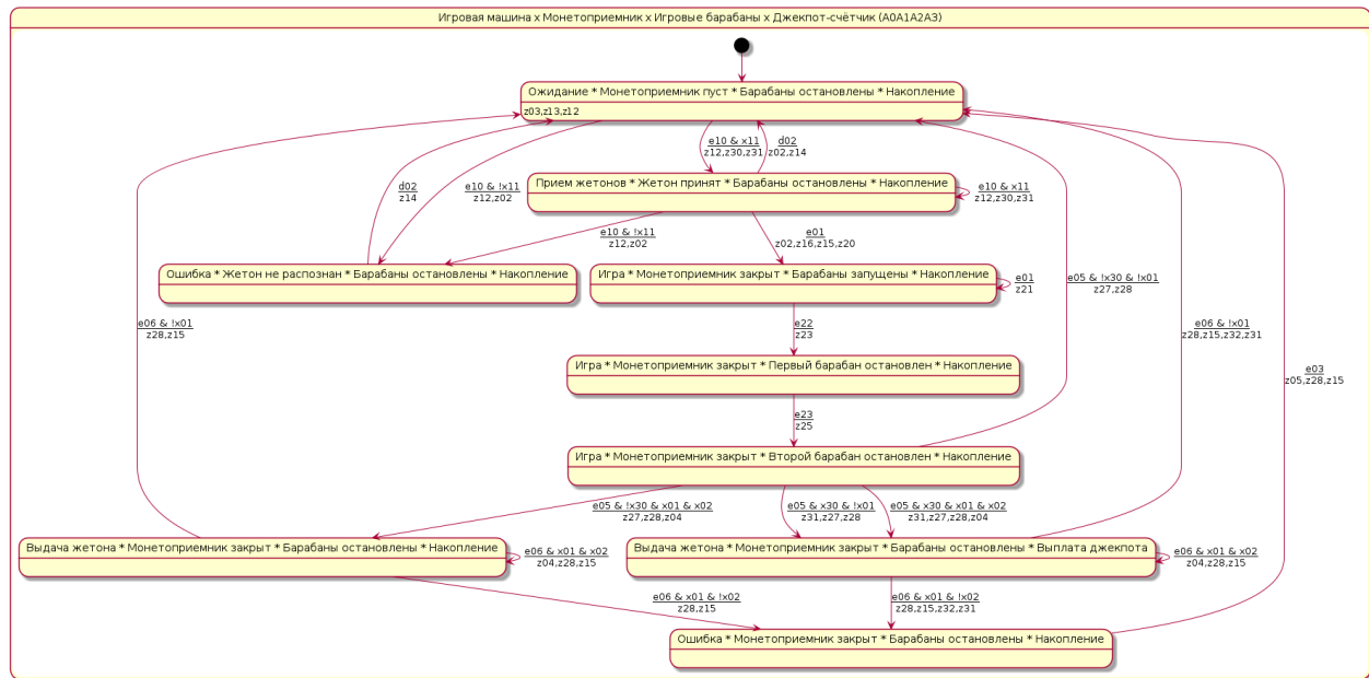
Рис. 5: Диаграмма состояний итогового автомата A_0 \times A_1 \times A_2 \times A_3 (PlantUML, из puml/final.puml ; 9 состояний).
