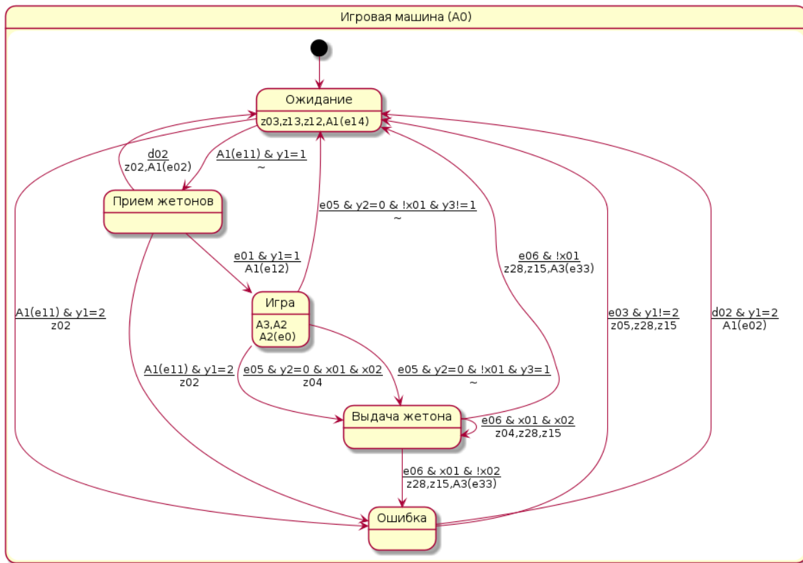
Рис. 1: Диаграмма состояний автомата A_0 (PlantUML, из puml/a0.puml ).
